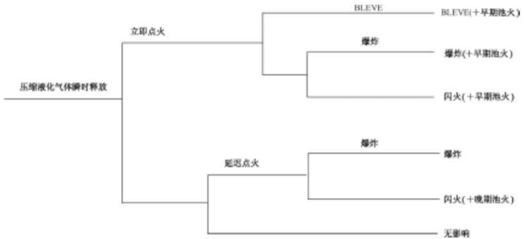
图 F.3 压缩液化气体瞬时释放事件树
