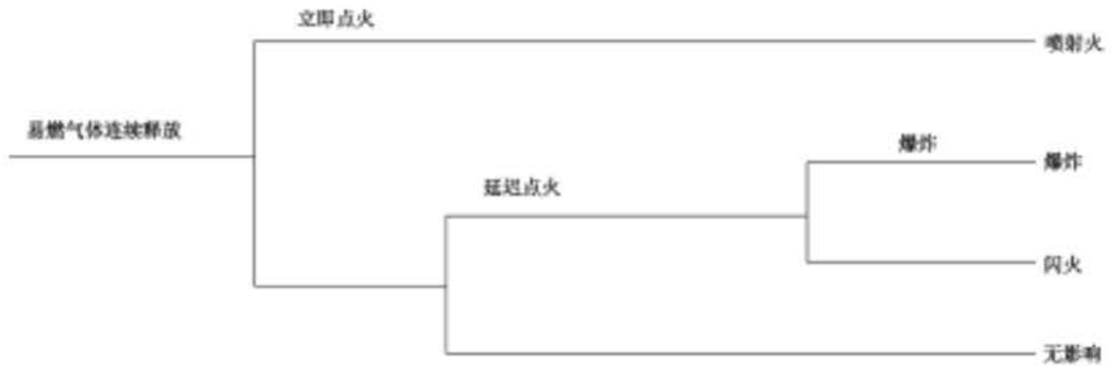
图 F.2 易燃气体连续释放事件树
