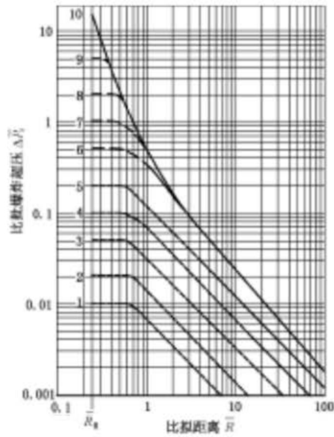
图 D.1 TNO 模型的 Sachs 比拟超压
