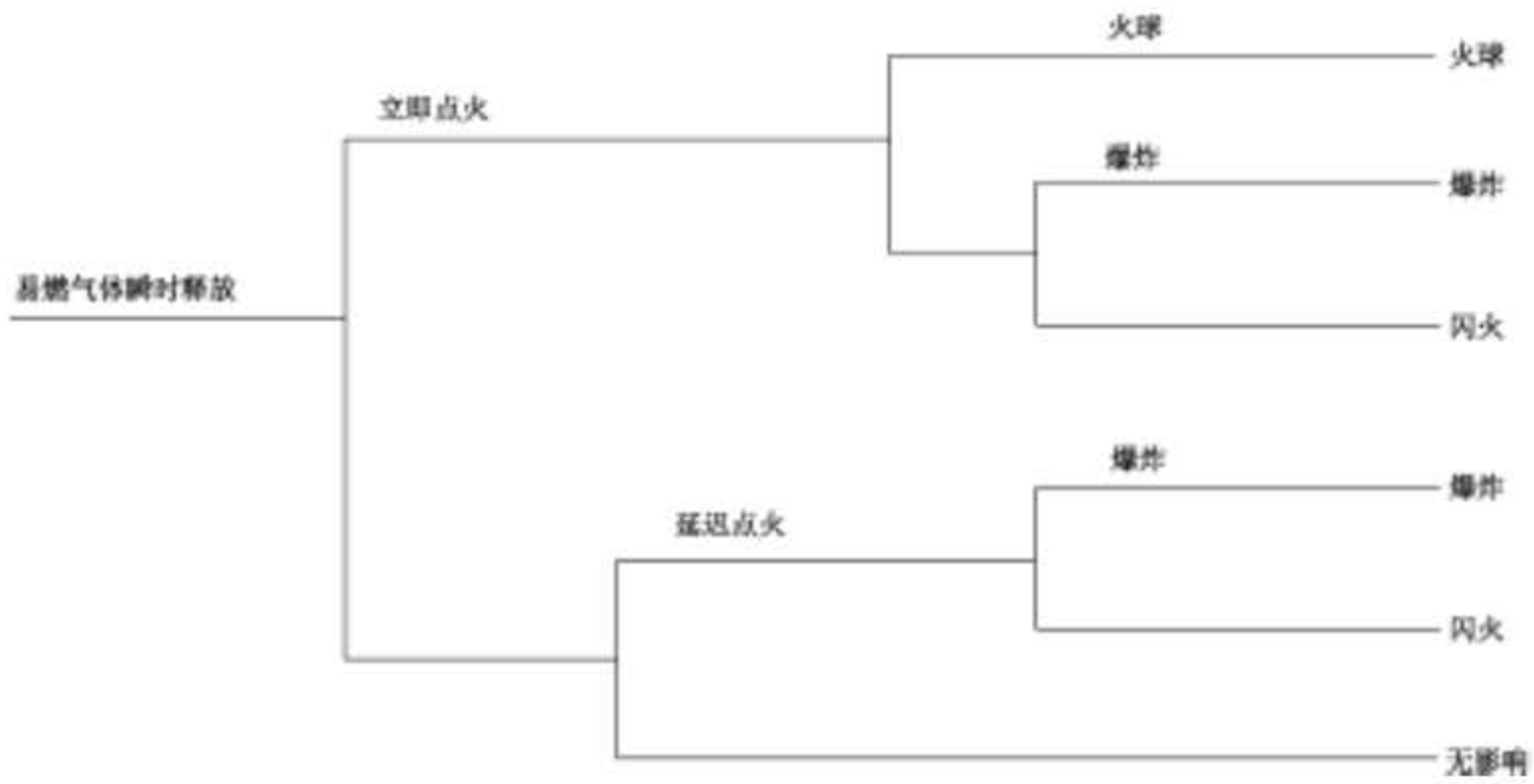
图 F.1 易燃气体瞬时释放事件树
