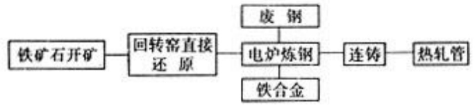
图3 直接还原-电炉流程(DRI/EAF)CO 2 排放边界
