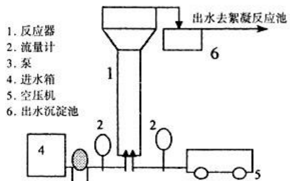
图 1 气升式生物膜反应器装置及流程示意图
