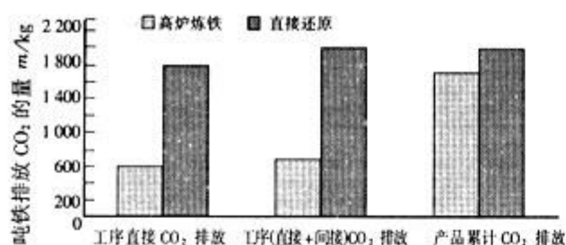
图4 几种流程的吨铁 CO 2 排放量比较
