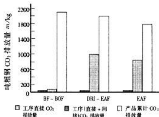
图5 几种流程的吨粗钢 CO 2 排放量比较
