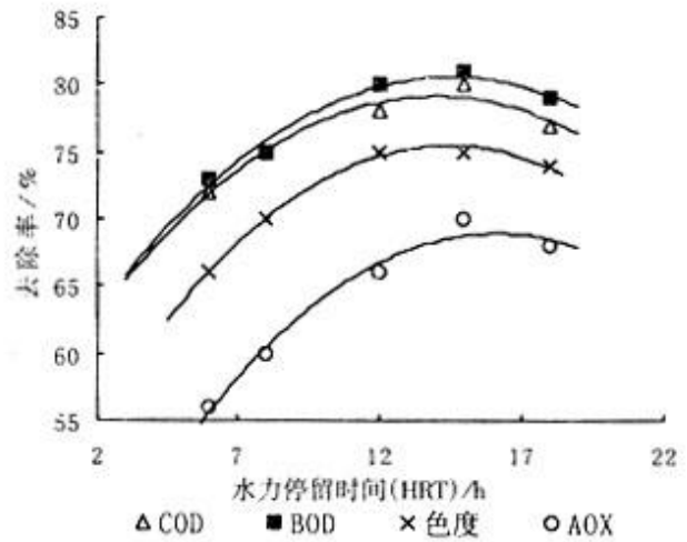
图5 不同HRT对几种污染物去除率的影响
