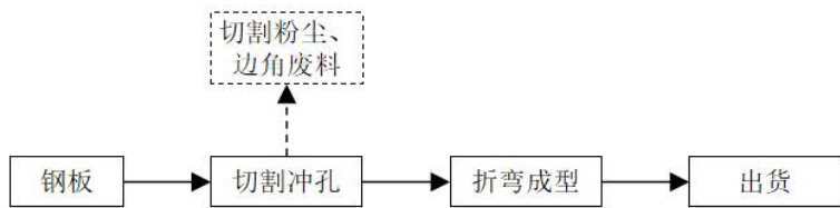
图 2-13 汽车零配件生产工艺流程及产污节点图
