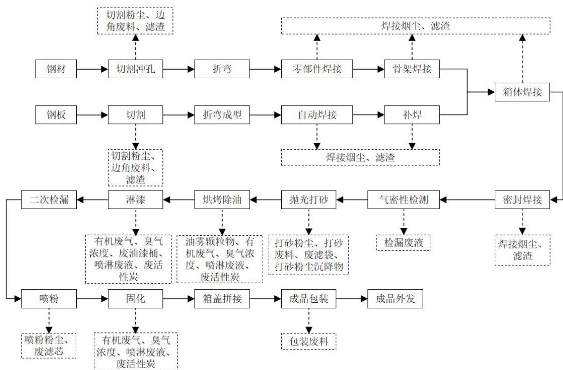
图 2-13 电压箱体生产工艺流程及产污节点图
