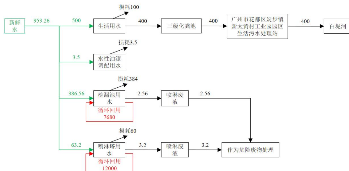
图 2-2 项目迁改建后近期水平衡图 (单位: t/a)
