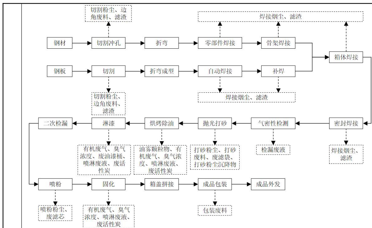
图 2-4 生产工艺流程及产污节点图
