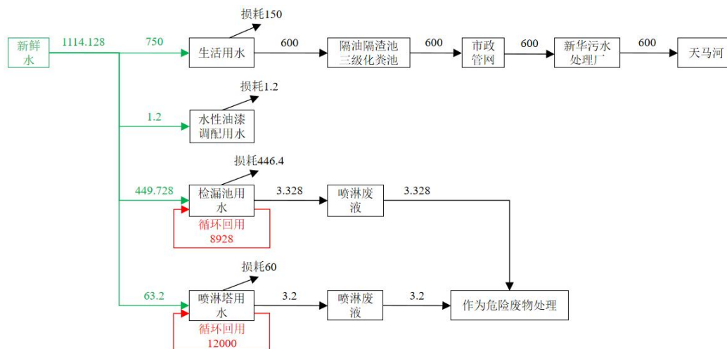
图 2-1 现有项目水平衡图 (单位: t/a)
