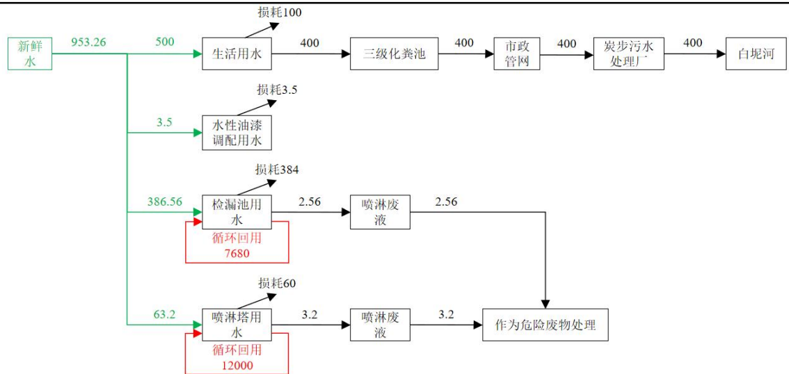
图 2-3 项目迁改建后远期期水平衡图 (单位: t/a)
