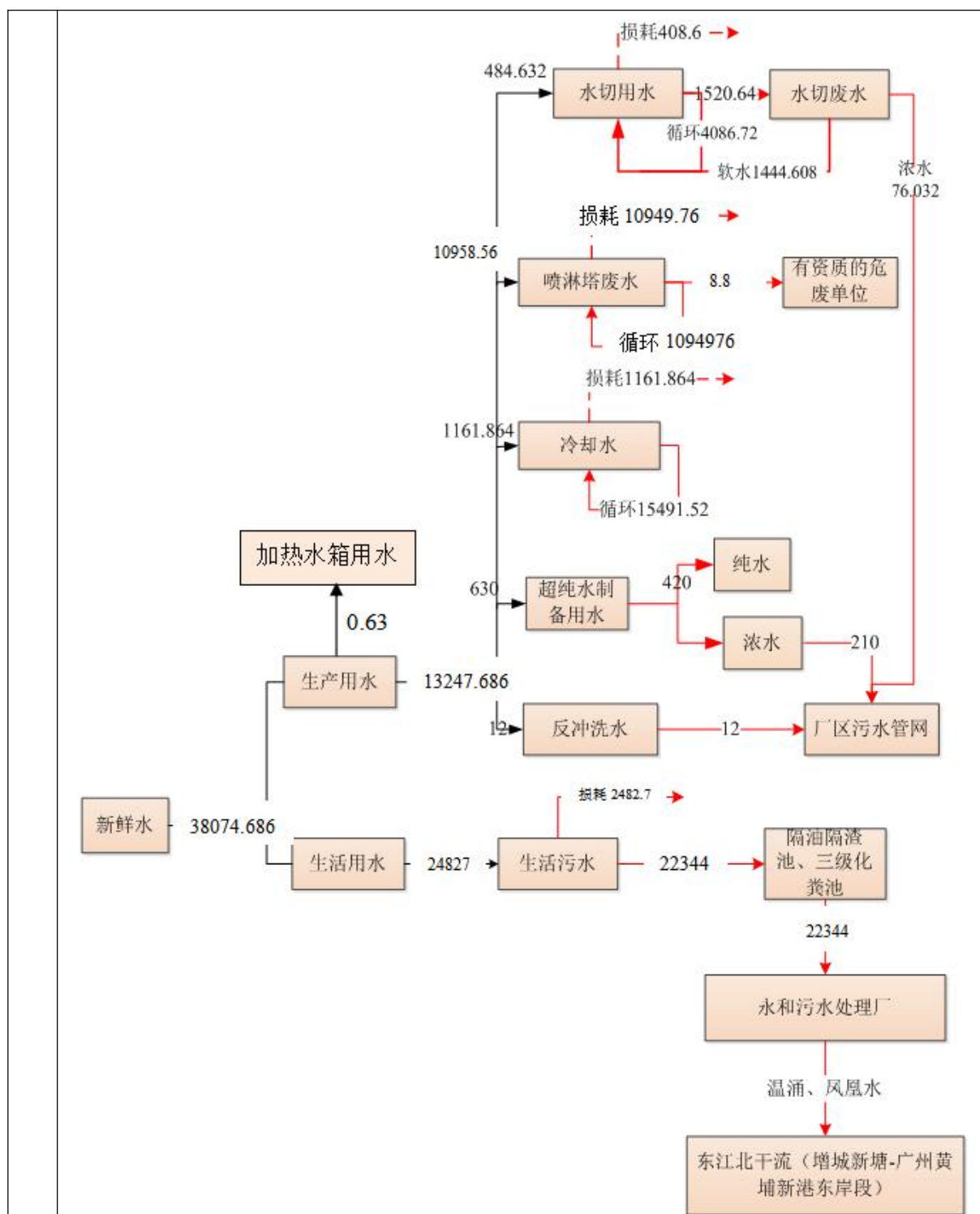
图 2-2 扩建后项目全厂水量平衡图 单位: t/a
