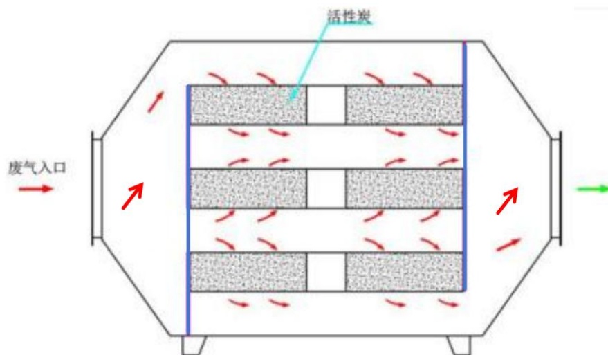
图 4-1 本项目活性炭箱设计图
