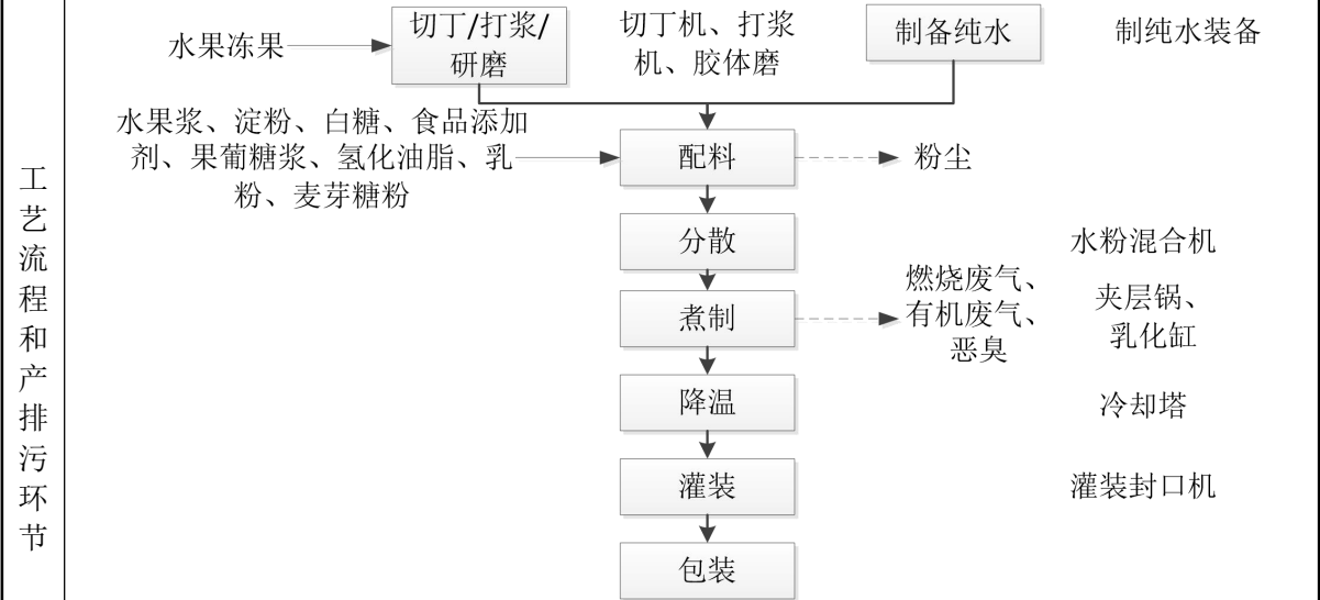
图 2-2 果馅、果茸和调味料生产工艺
