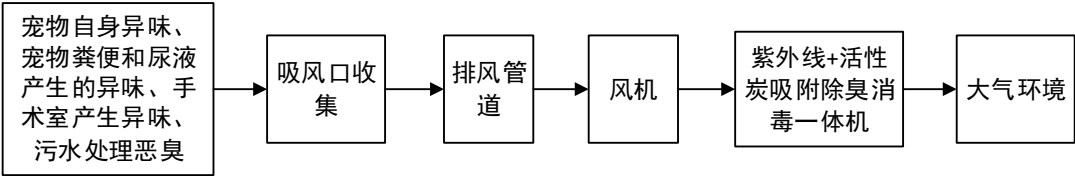
图 4 项目废气处理工艺流程图
