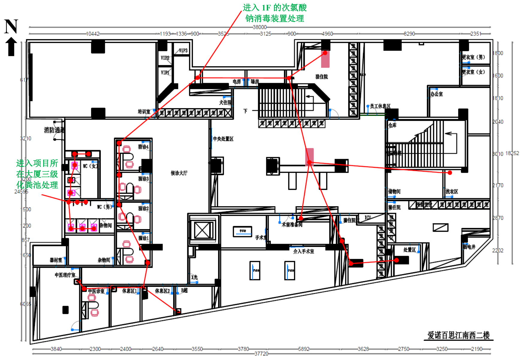
附图 9 项目 2F 排水图
