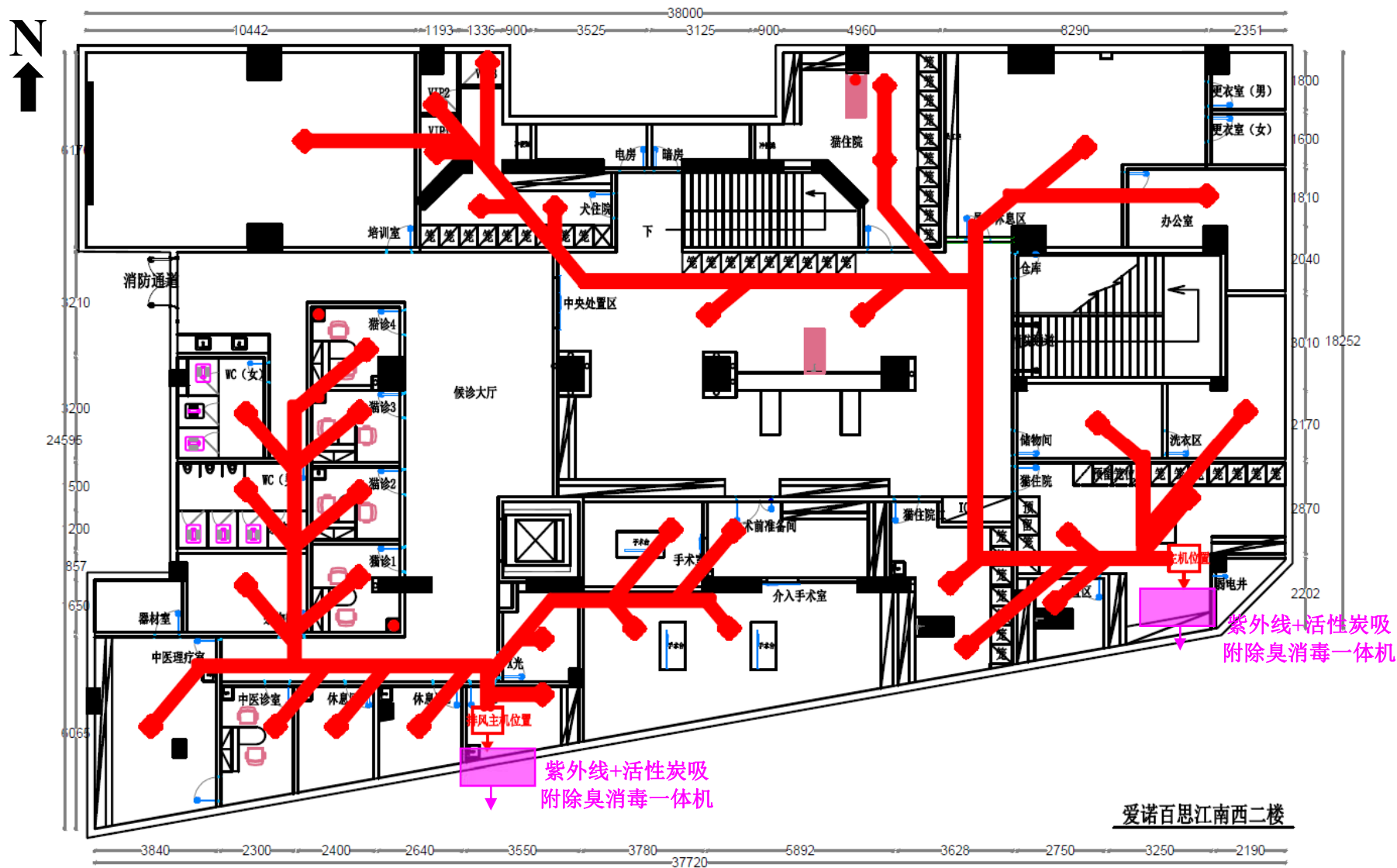
附图 7 项目 2F 排风图
