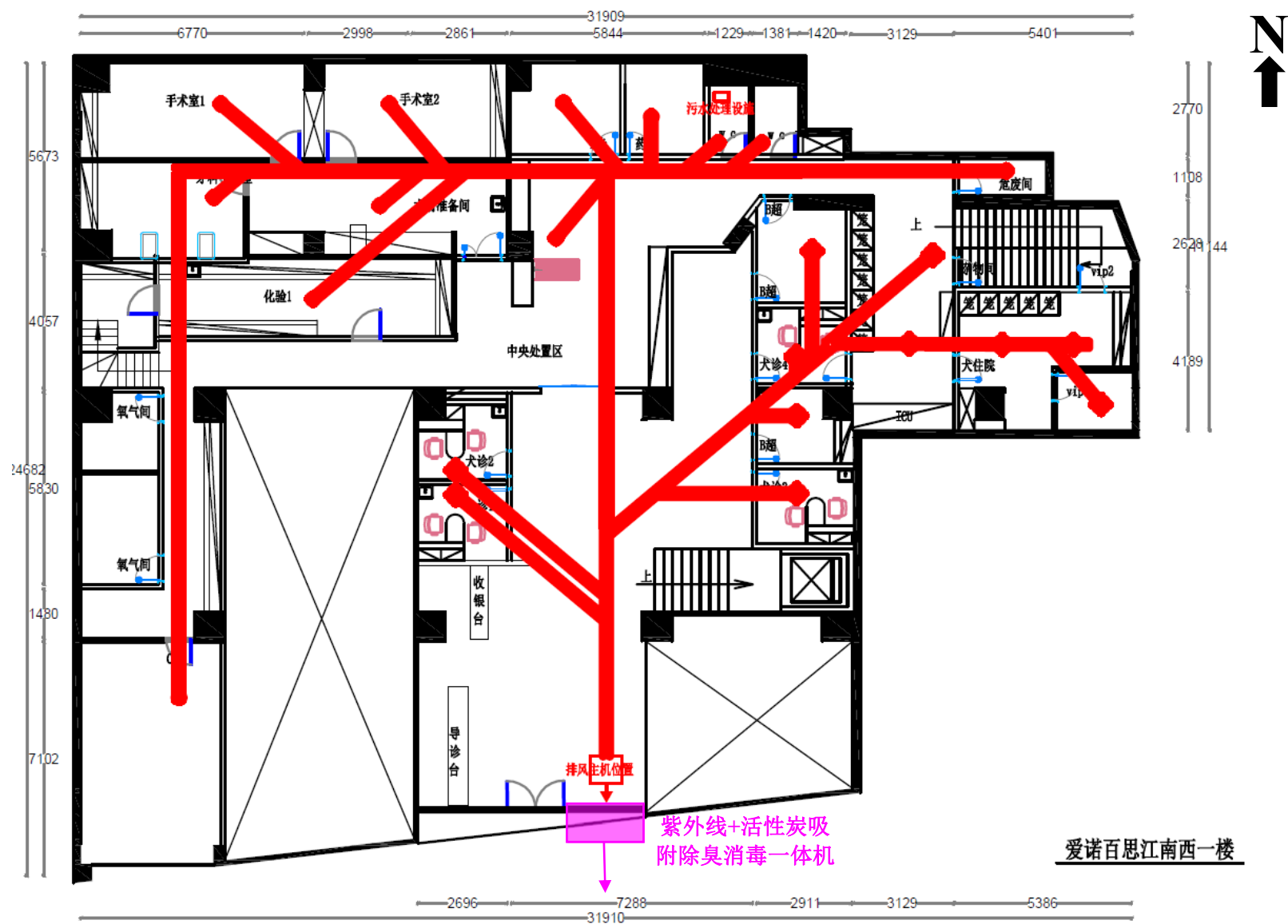
附图 6 项目 1F 排风图
