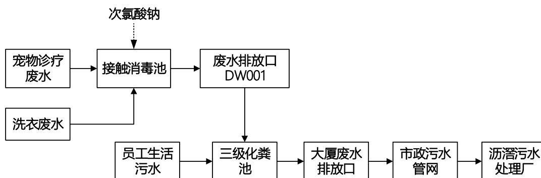
图7 本项目废水处理工艺流程图
