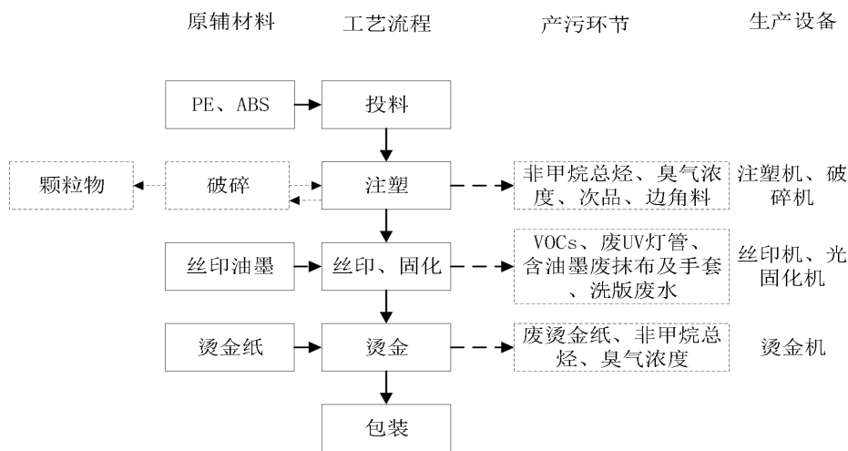
图 2-2 化妆瓶生产工艺流程图
