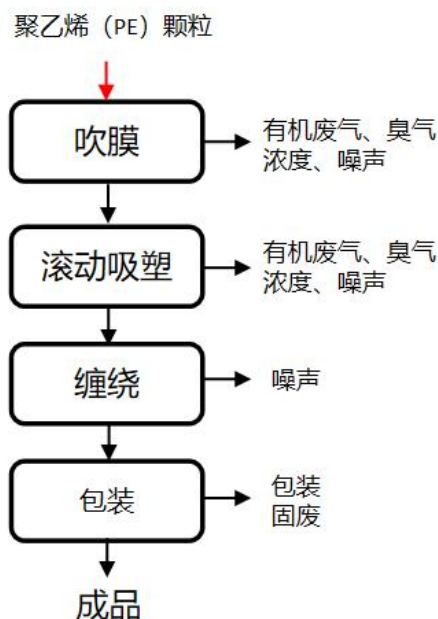
图 2-2 塑料气泡膜生产工艺流程及产污环节图
