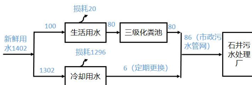
图 2-1 本项目水平衡图 (t/a)
