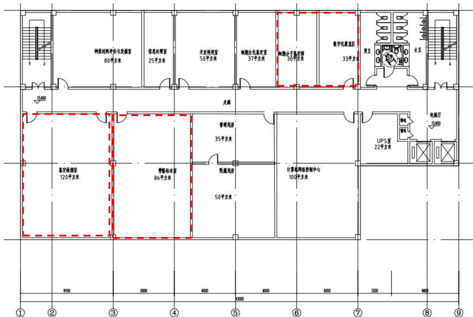
附图 4-5 5 楼平面布置图
