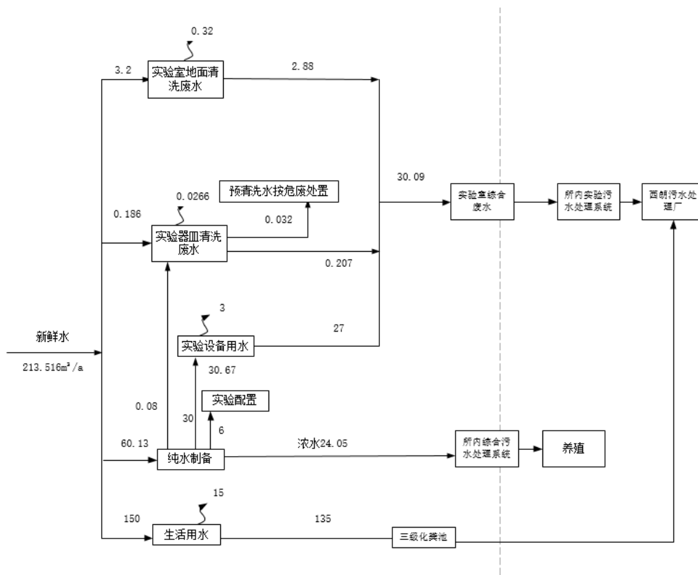
项目水平衡图 (m³/a)
