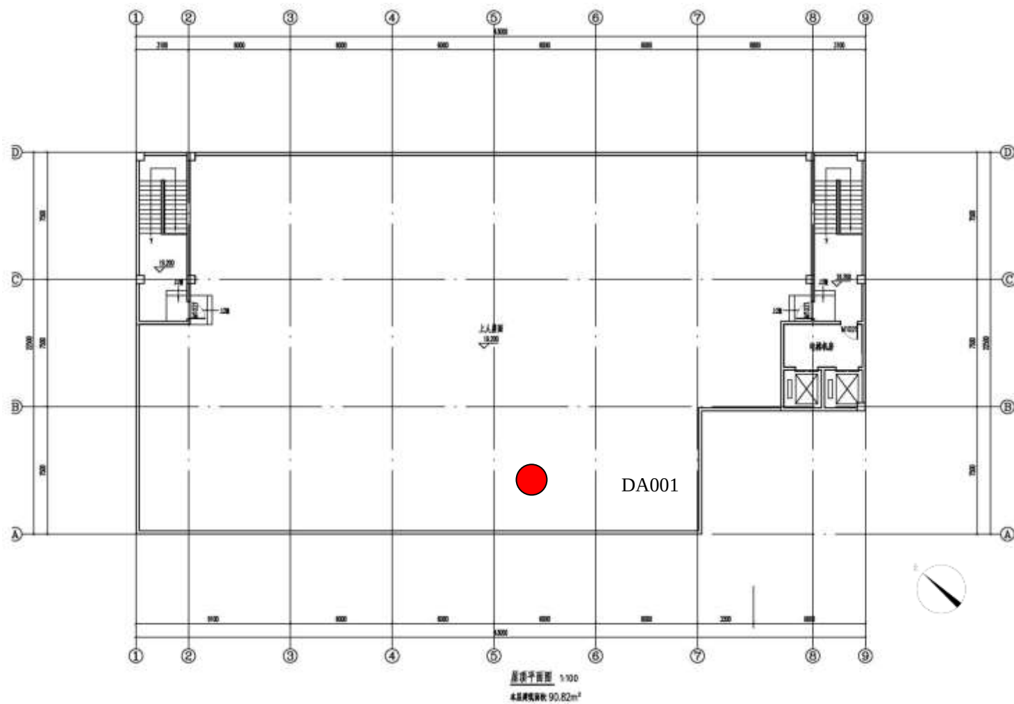
附图 4-6 顶层平面布置图
