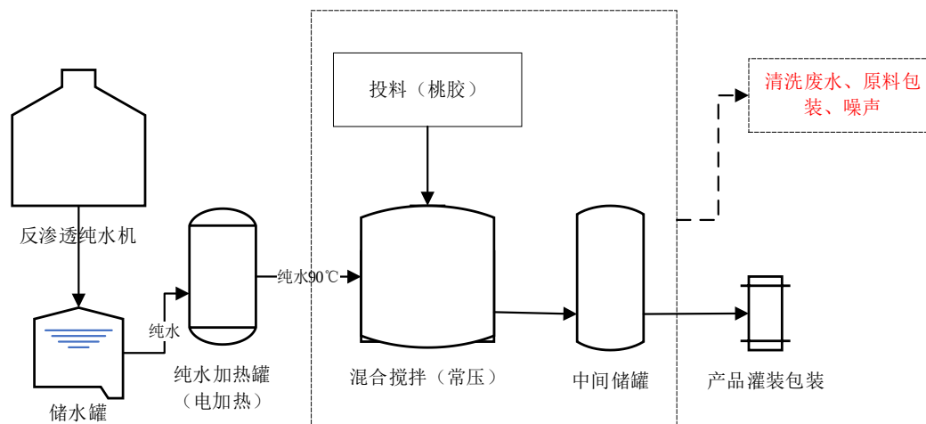
图 2-5 保护胶生产工艺流程及产污环节
