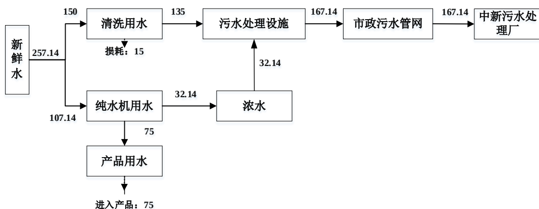
图 2-1 本次改扩建用水水平衡图 单位 \text{m}^3/\text{a}
