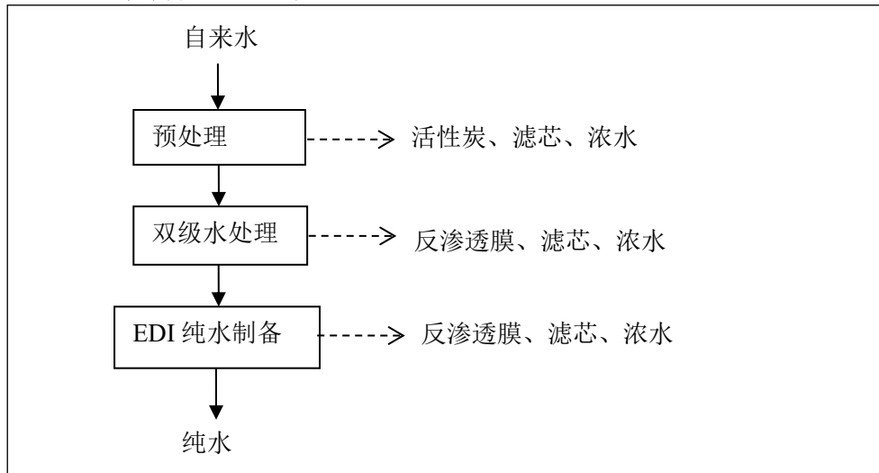
图 2-6 纯水制备工艺流程及产污环节
