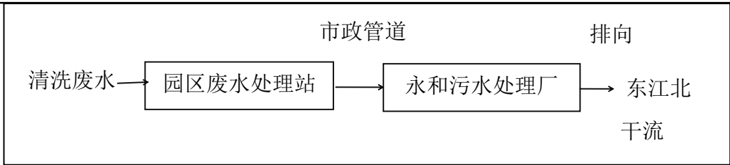
图 4-2 项目清洗废水处理工程流程图
