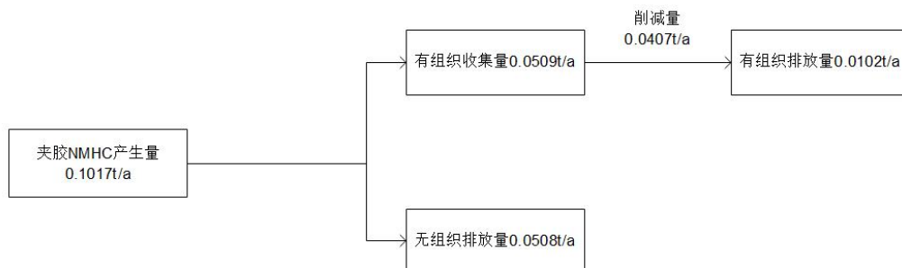
图 4-2 项目有机废气平衡图
