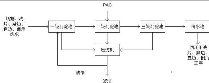
图 4-1 污水处理设施处理流程
