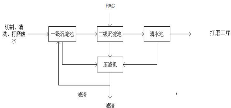
图 4-1 污水处理设施处理流程
