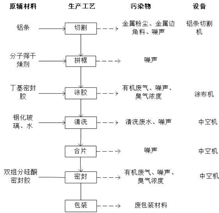
图 2-3 中空玻璃生产工艺流程
