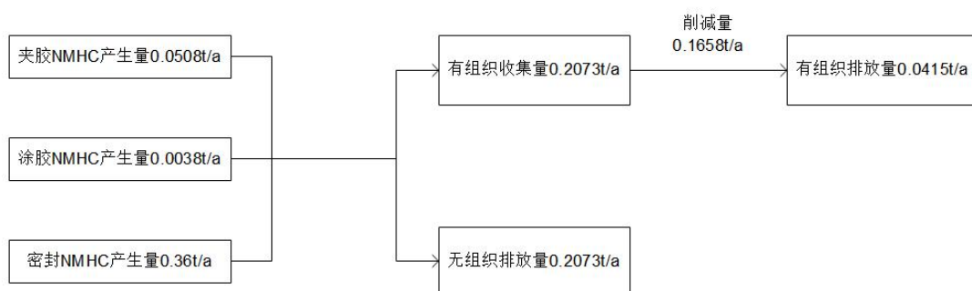
图 4-2 项目有机废气平衡图
