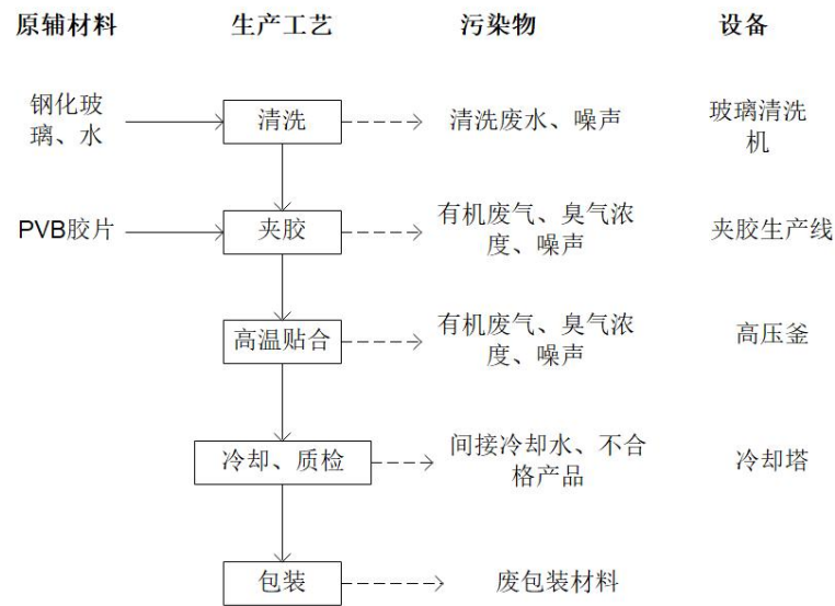
图 2-4 夹胶玻璃生产工艺流程
