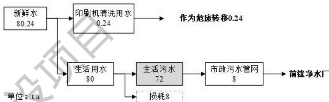
图 2-1 水平衡示意图
