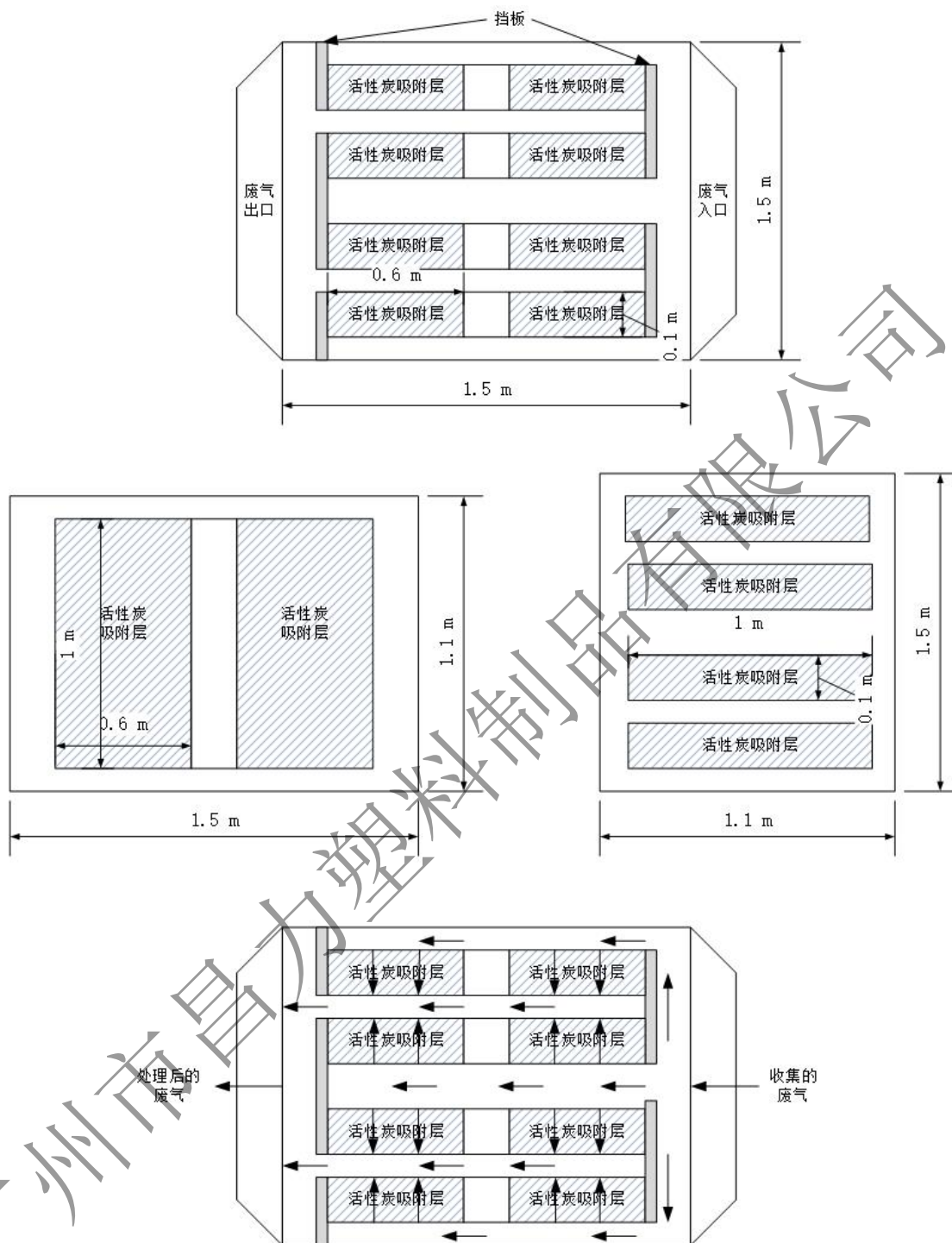
图 4-1-1 活性炭吸附器（第一级）内部结构和气流走向示意图
