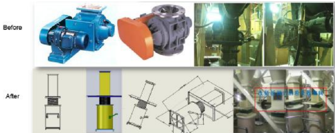
图 改进部件示意图
