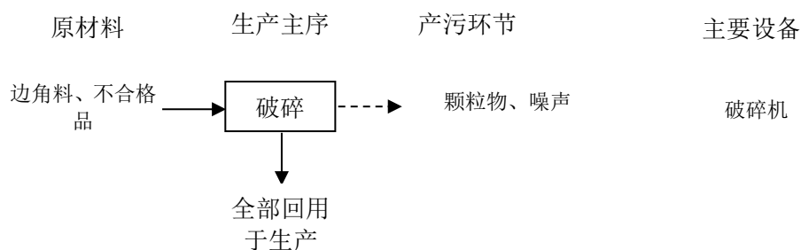
图 2-4 本项目破碎工艺流程及产排污环节图
