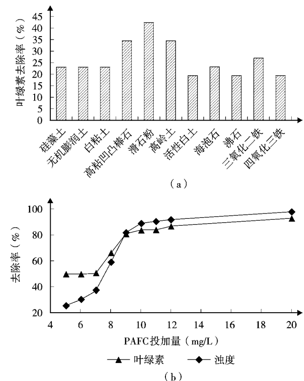
图 1 不同种类粘土以及 PAFC 单独投加对叶绿素的去除率
