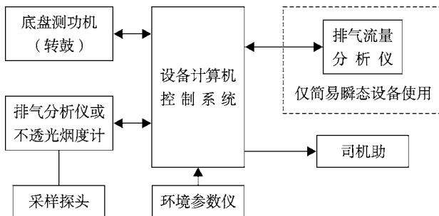
图 1 简易工况法设备构成
