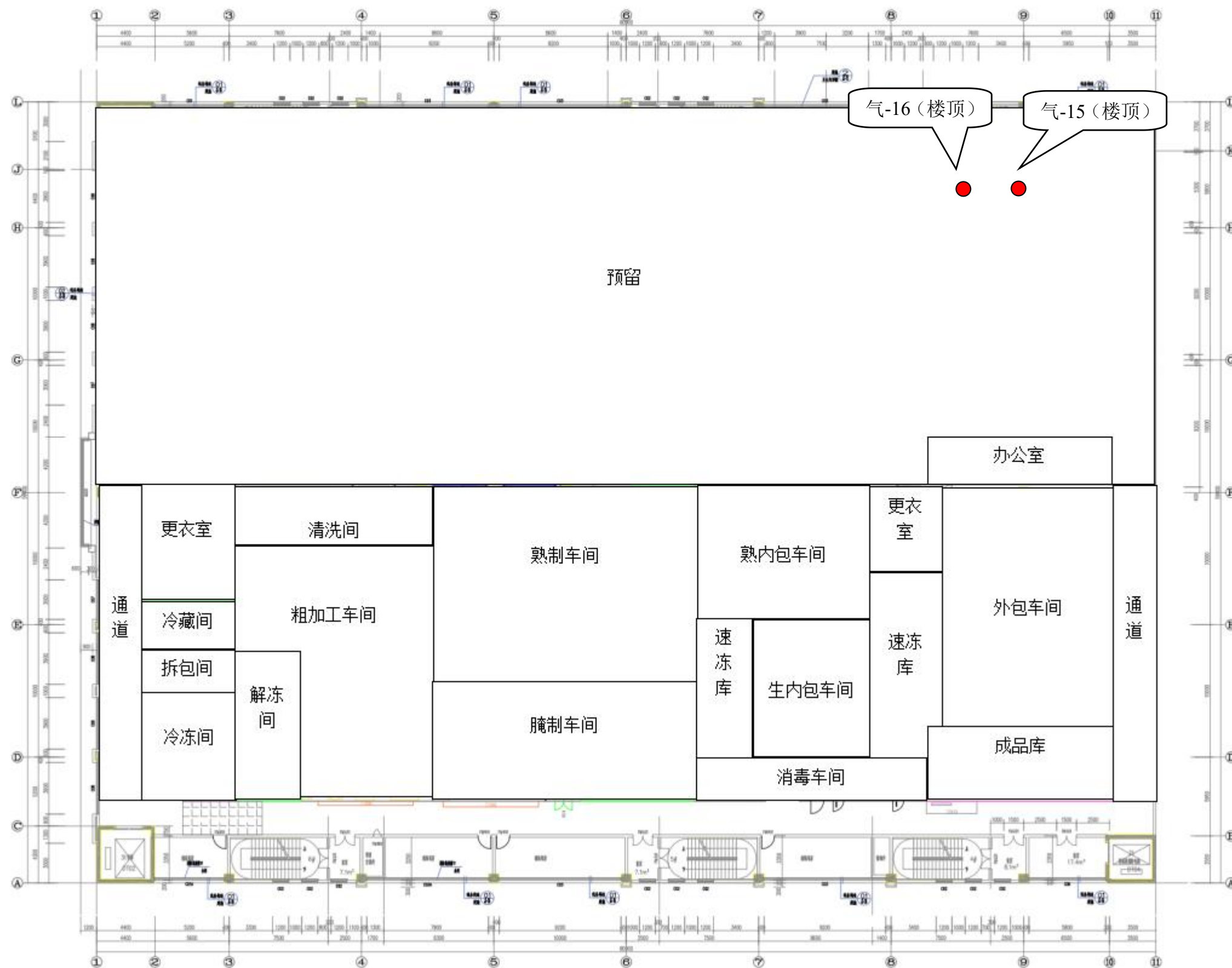
附图 3 本项目平面布局图
