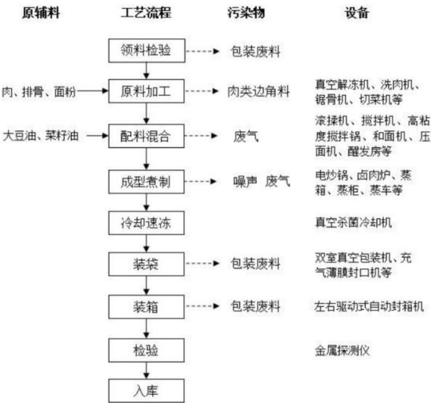
图2-9马拉糕、流沙包、馒头、过水鸭头、排骨串工艺流程图
