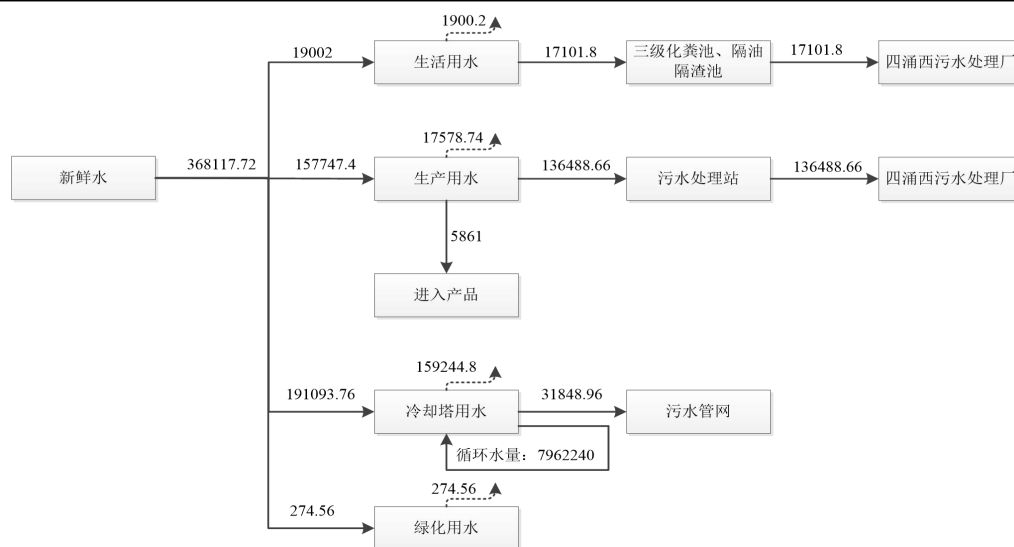
图 2-3 扩建后全厂项目水平衡图 (单位: t/a)
