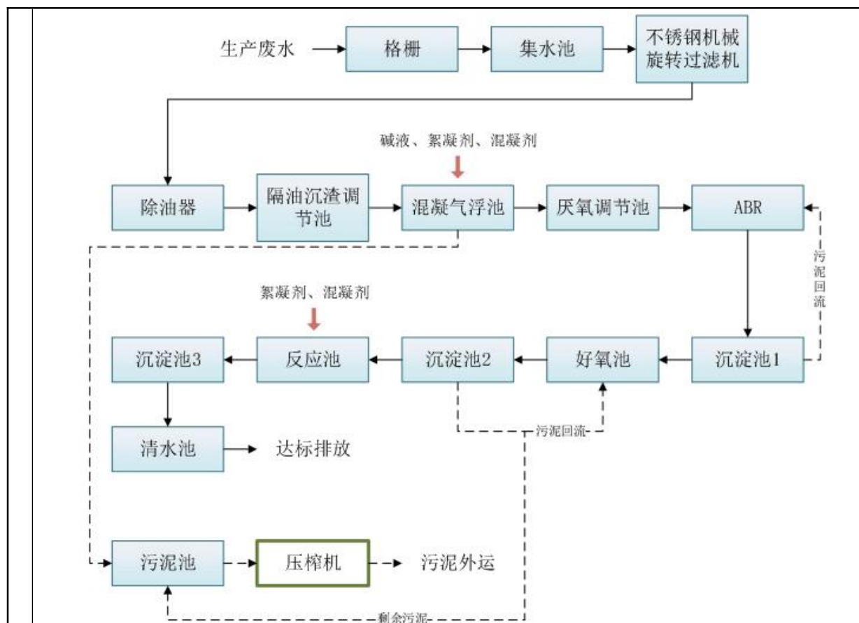
图 4-1 生产废水处理工艺流程图
