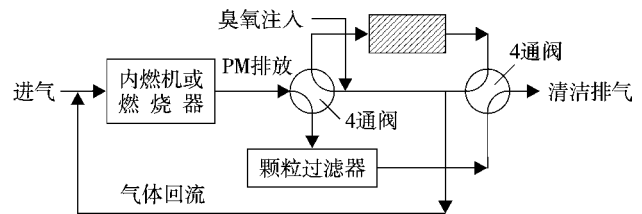
图 1 \text{O}_3 氧化碳烟装置示意
