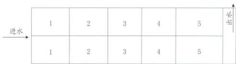
图4-4 广州市番禺东涌工业污水处理有限公司四期活性污泥处理流程图
