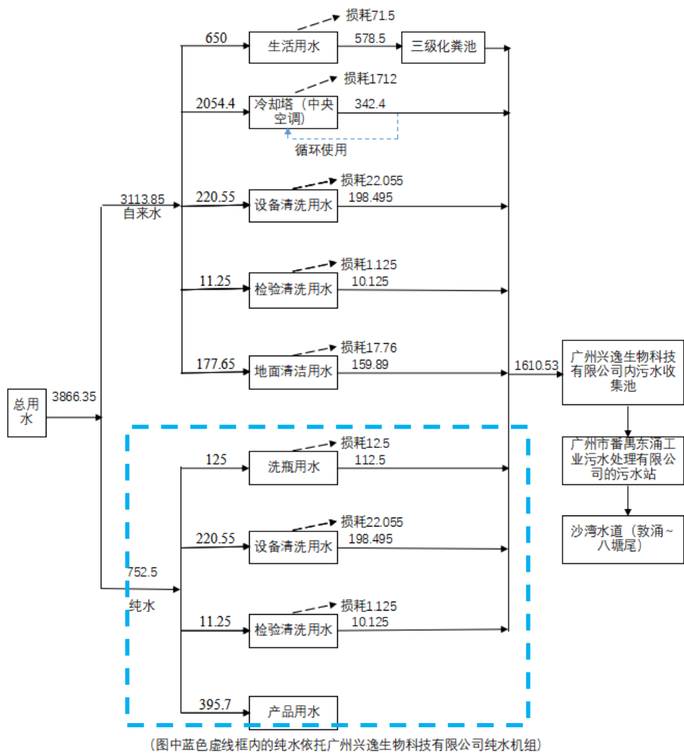
图 2-2 改建项目水平衡图 单位: \text{m}^3/\text{a}
