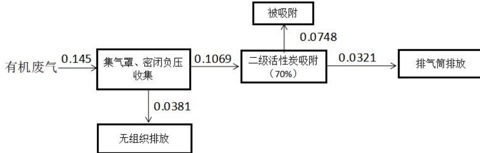
图 4-1 项目有机废气平衡图 (t/a)
