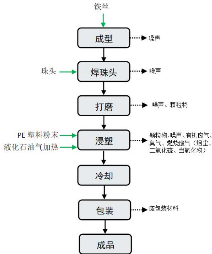
图2-2 衣架生产工艺流程图
