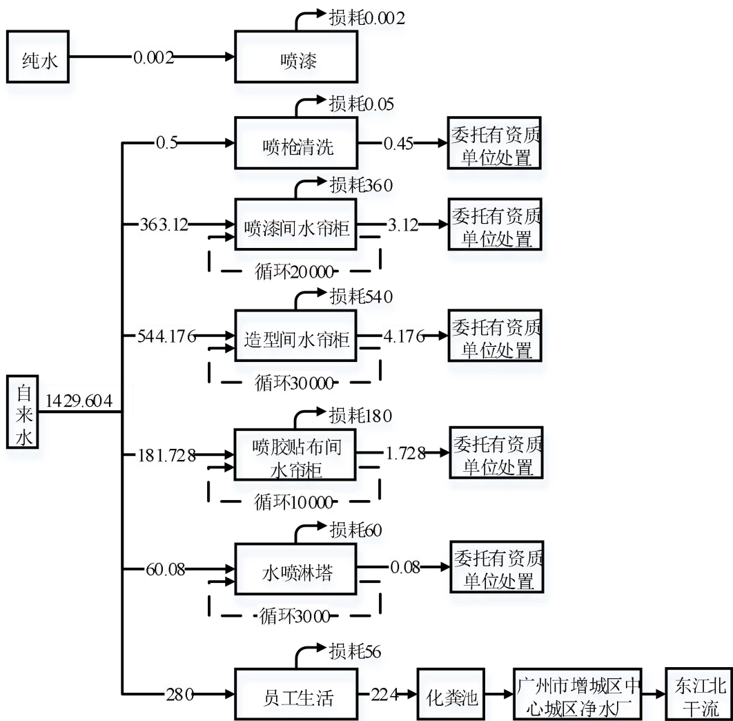
图2-2 本项目水平衡图，单位m³/a
