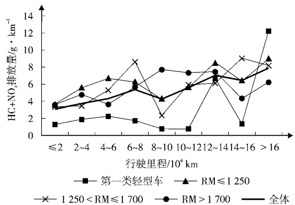
图4 各行驶里程车辆HC+NO x 排放均值
