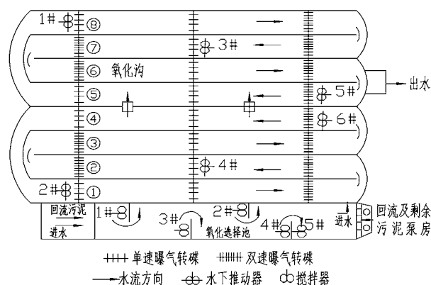
图 1 改良氧化沟单组沟平面示意
