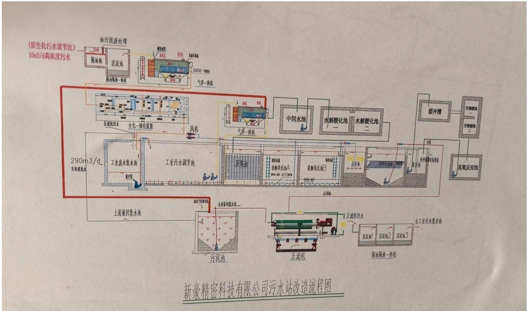
附图 3-7 新豪公司污水处理站工艺流程图
