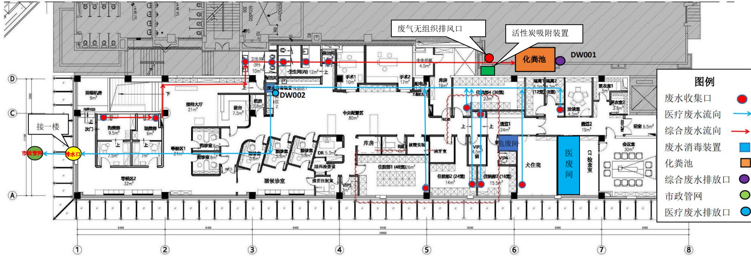
附图 4-3 项目平面布置图-排水图
