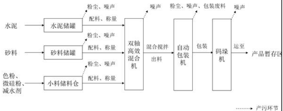
图 2-1 项目生产工艺流程图
