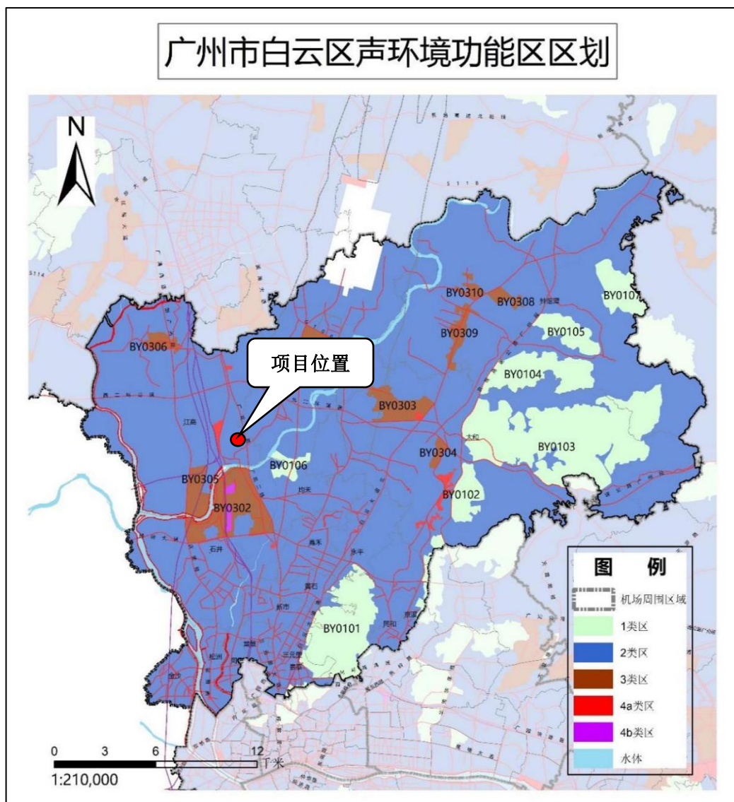
附图7 广州市声环境功能区划（2类区）
