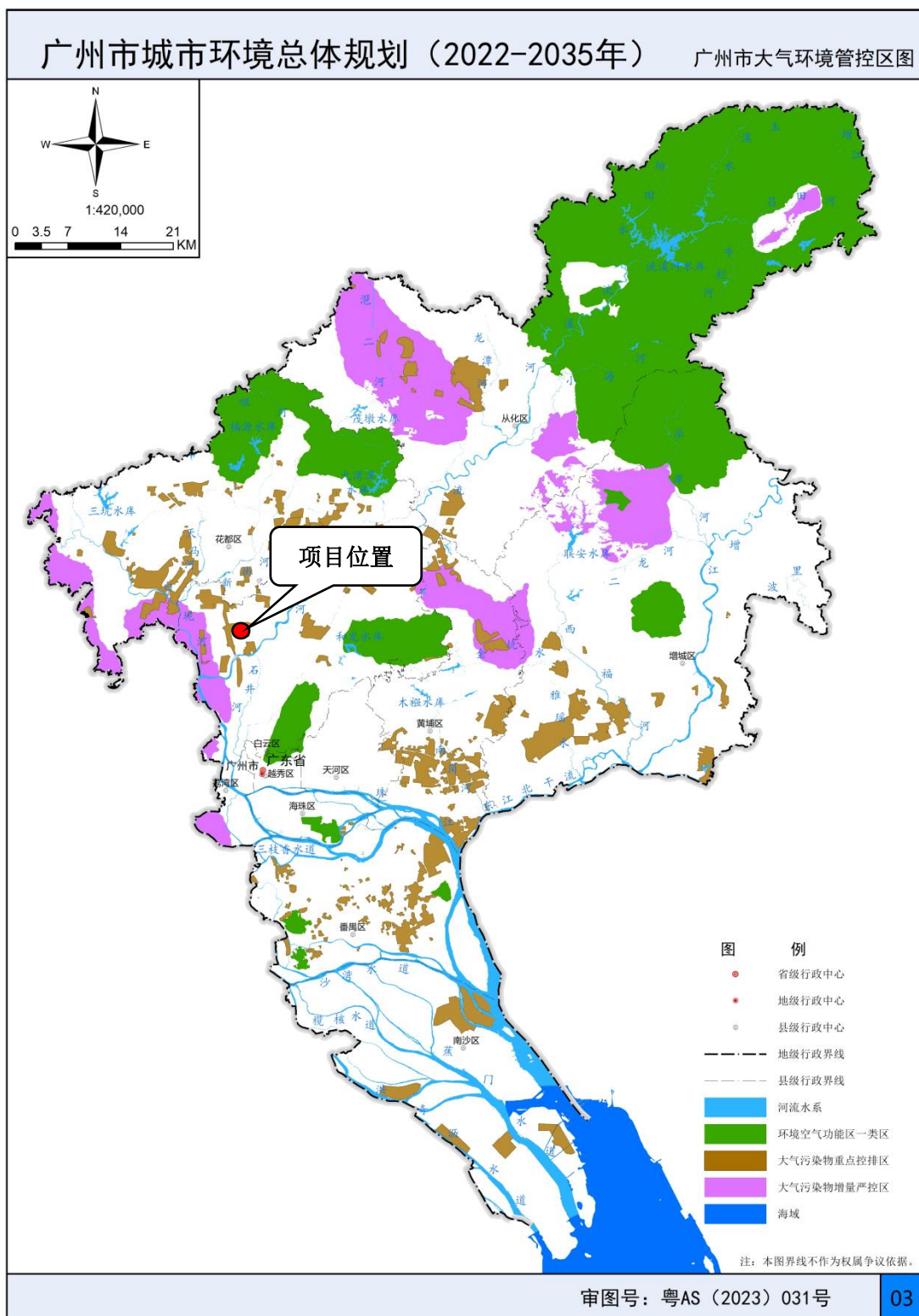
附图9 广州市大气环境空间管控区图
