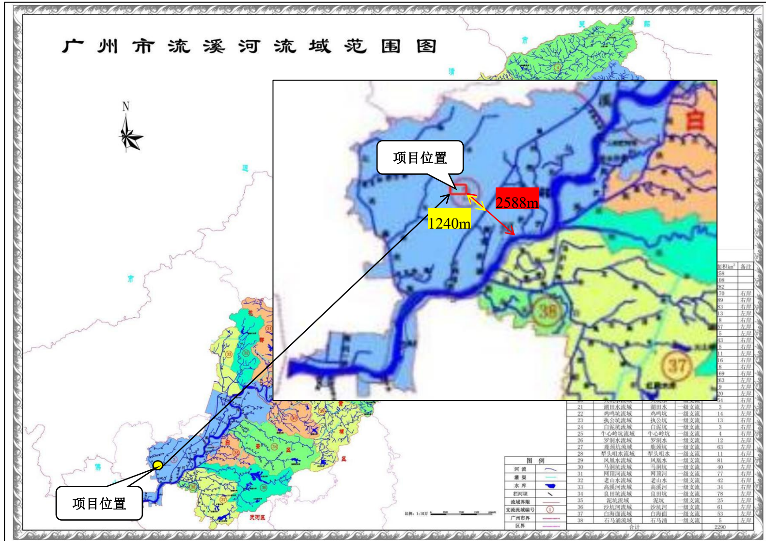
附图14 广州市流溪河流域水系图
