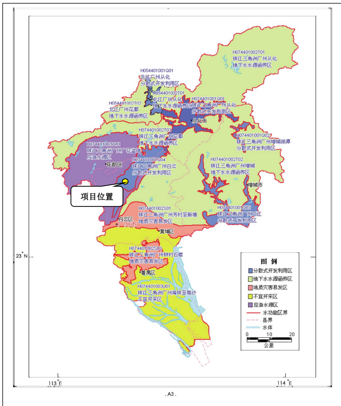
附图 13 项目所在地浅层地下水环境功能区划图
