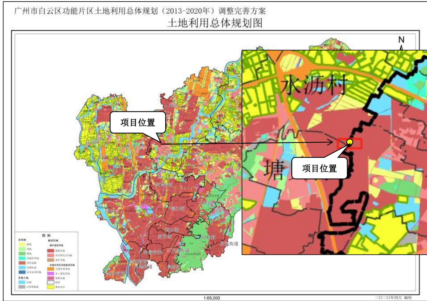
附图15 白云区土地利用总体规划图（2013-2020年）
