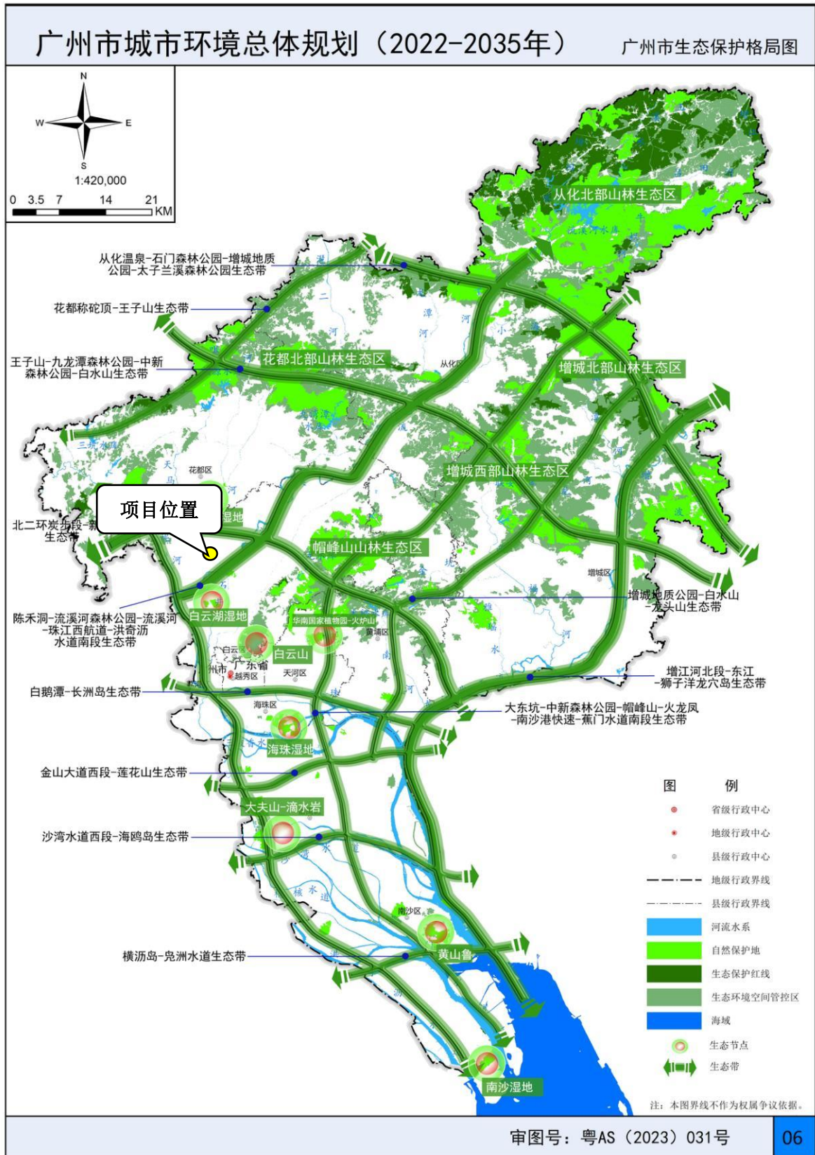
附图 8 广州市生态保护格局图
