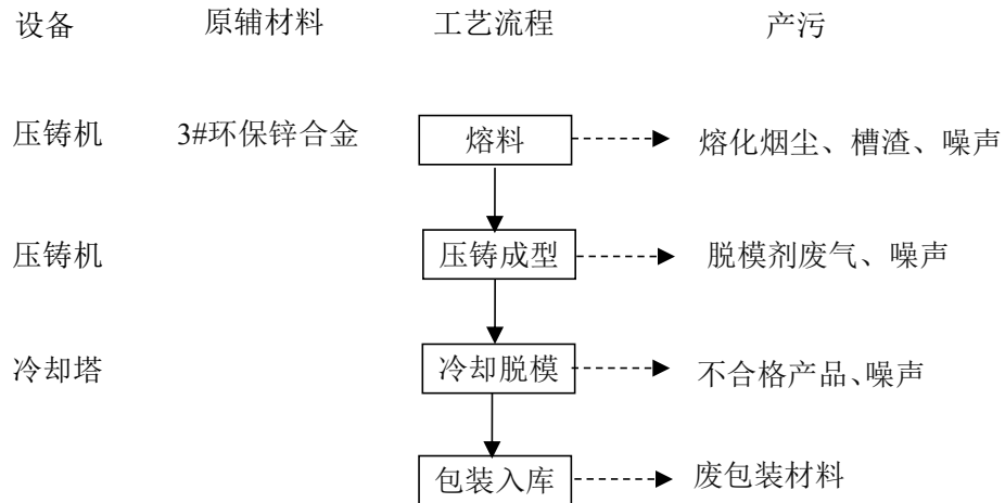
图 2-2 项目生产工艺流程及产污环节图
