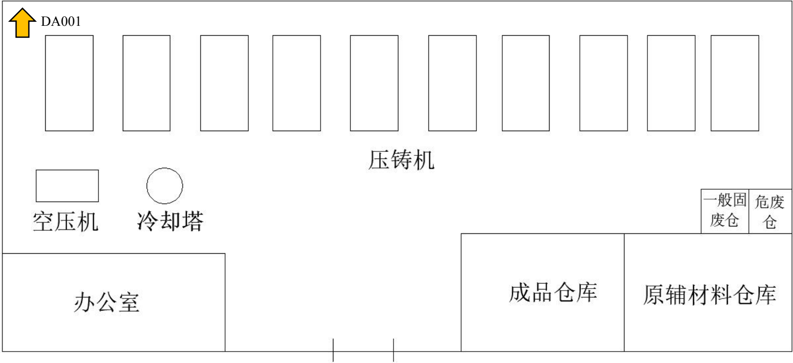
附图 5 项目平面布局图
