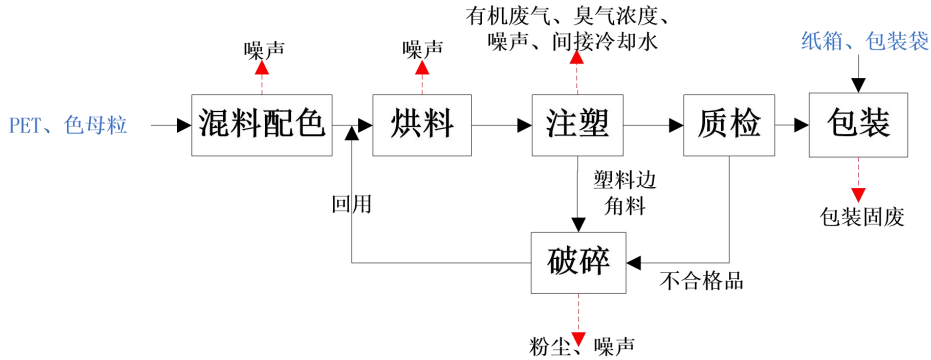
图 2-3 PET 瓶胚生产工艺流程及产污节点图
