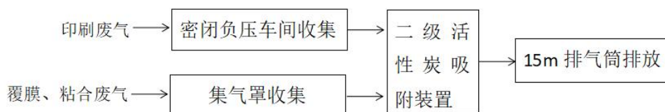
图 4-2 废气处理工艺图
