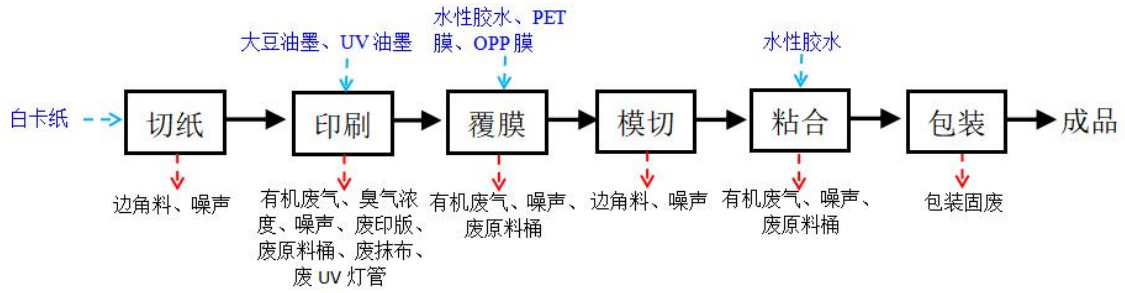
图 2-2 化妆品彩盒生产工艺流程及产污环节图
