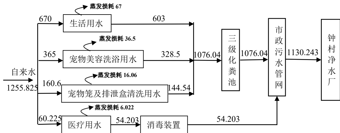
图 2-2 扩建后整体项目水平衡图 (单位: m 3 /a)
