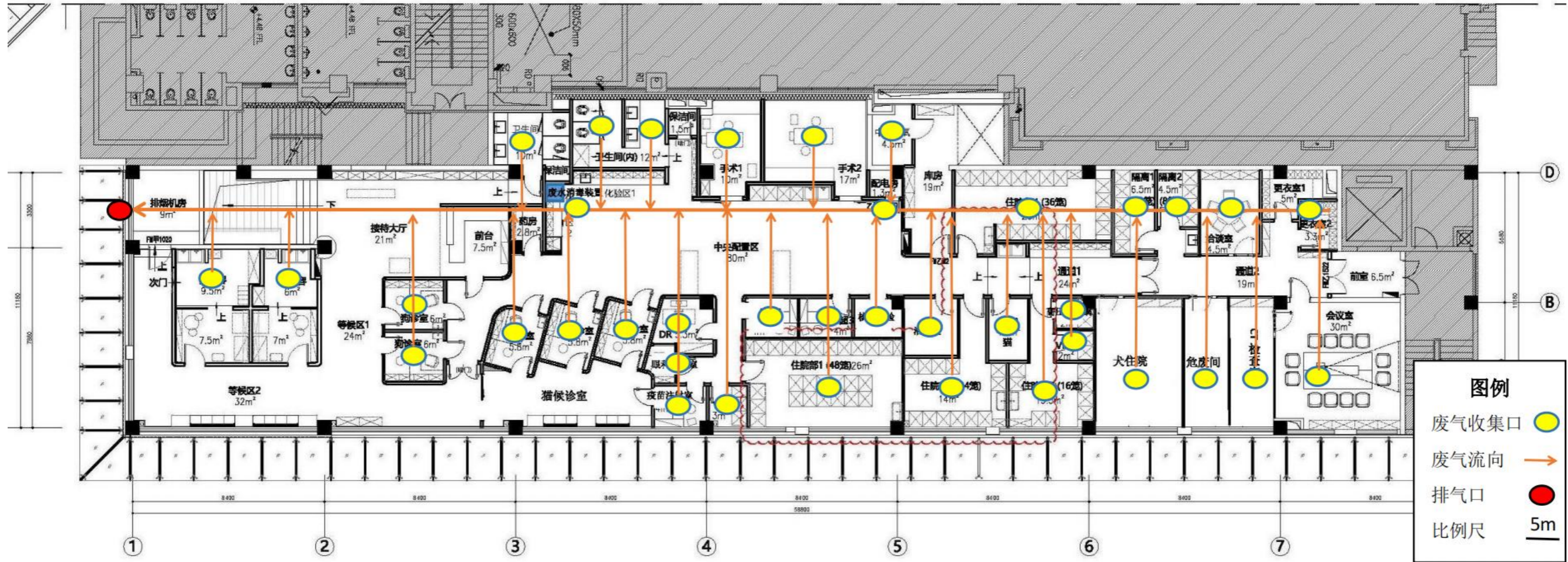
附图 4-2 项目平面布置图-排气图
