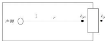
图 4-1 室内声源等效为室外声源图例
