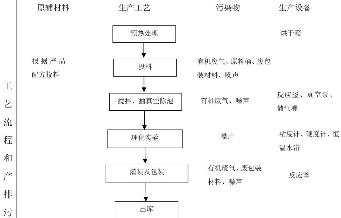
图 2-1 密封胶 A 胶、密封胶 B 胶生产工艺流程及产污节点图
