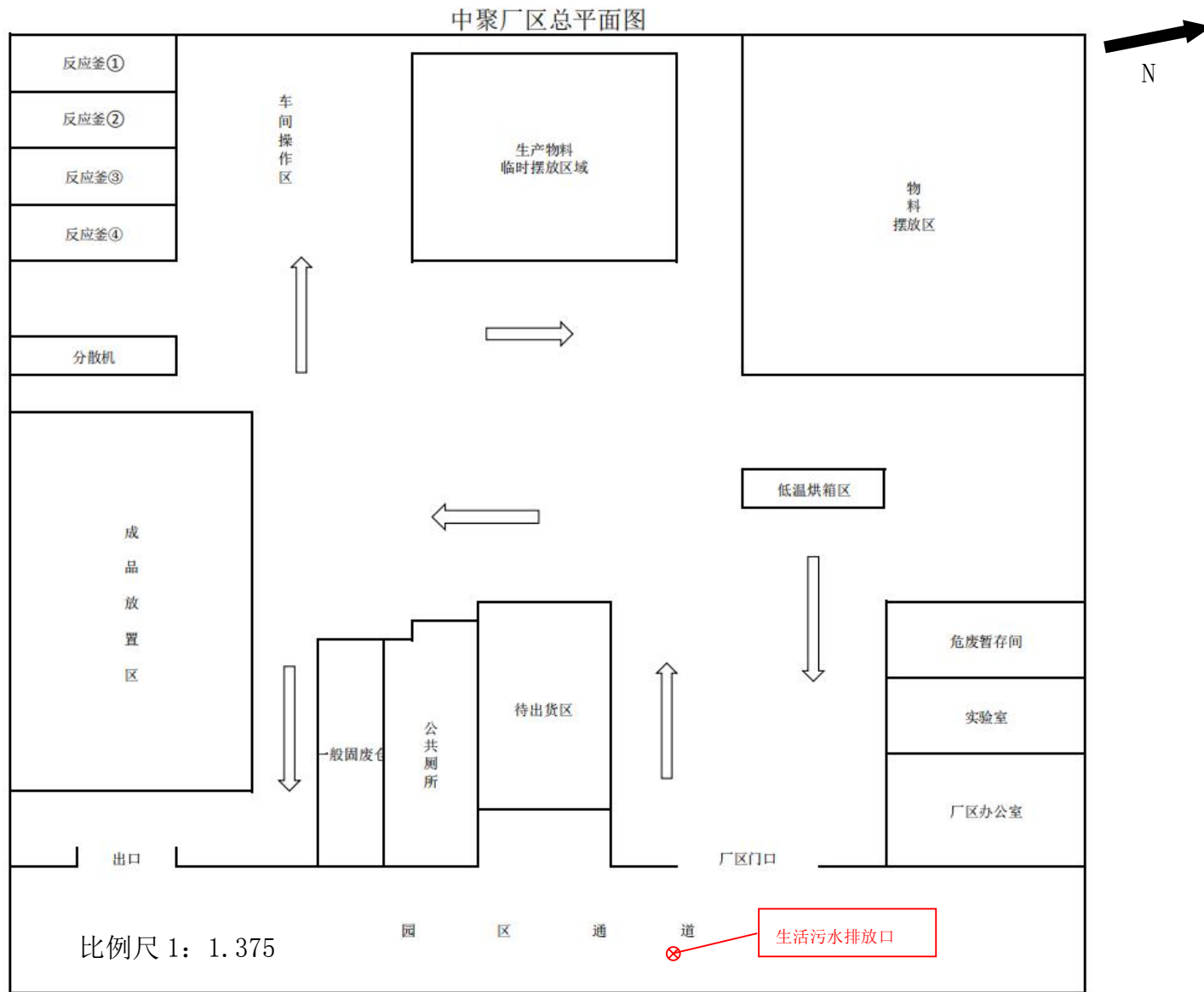
附图 3 项目厂区平面布置图
