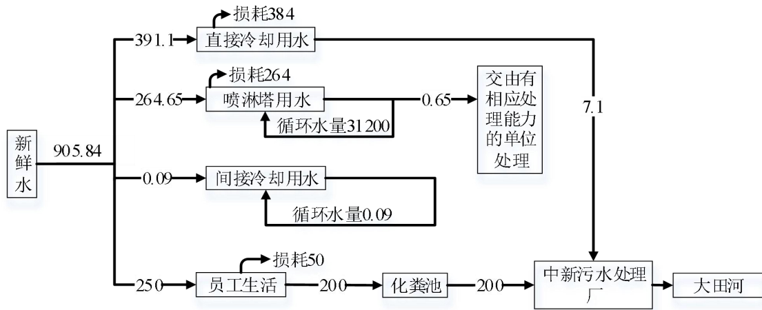
图2-2 本项目水平衡图，单位m 3 /a
