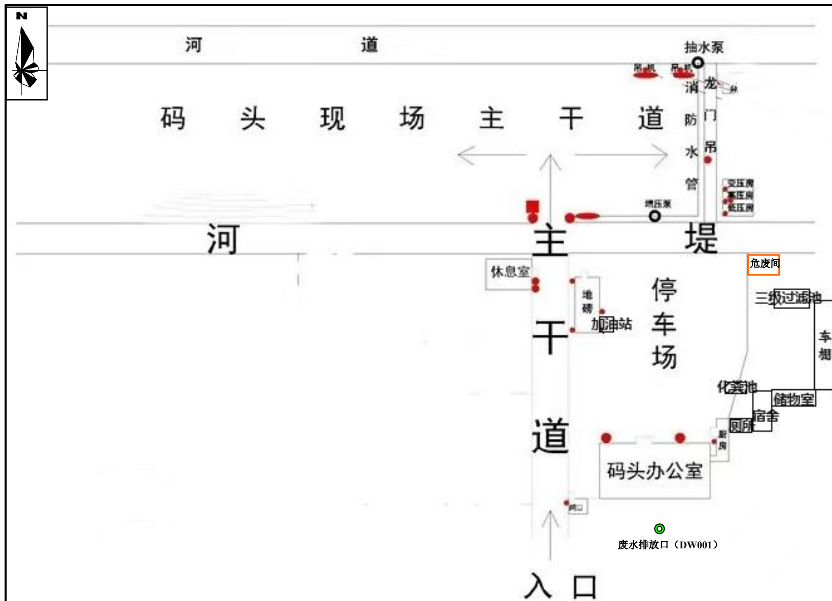
附图 5 (a) 项目码头总体平面布置图
