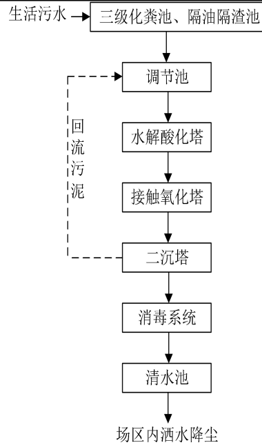
图 4-1 生活污水处理工艺流程图
