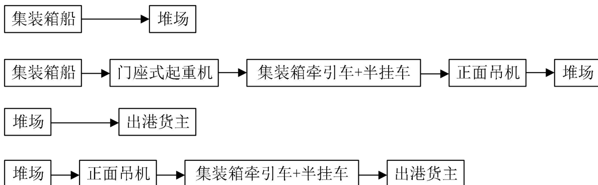
图 2-3 集装箱卸船流程图
