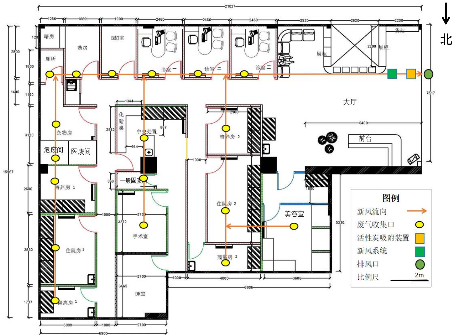
附图 4-1 项目平面布置图-废气流向
