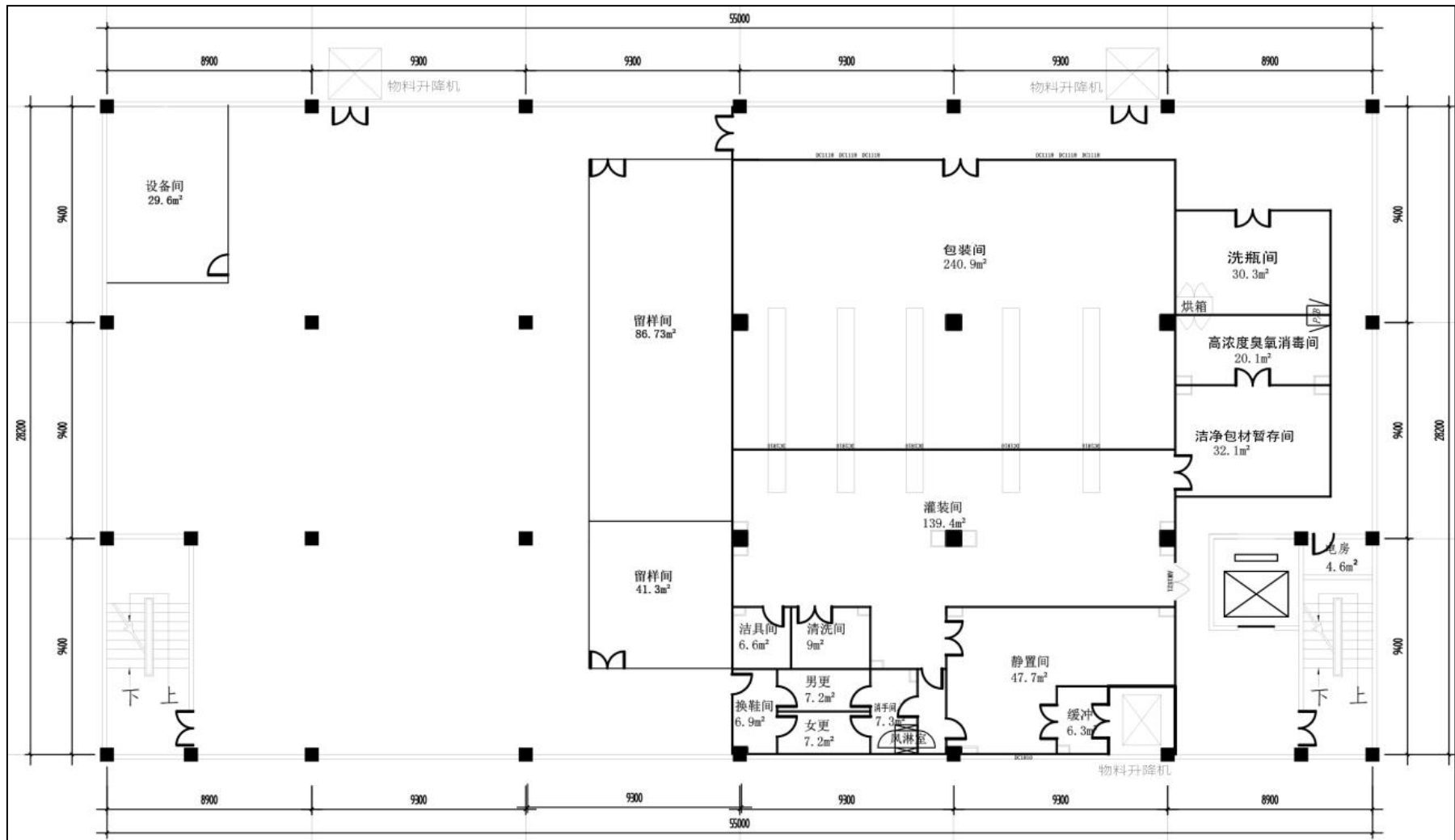
附图 5-2 扩建项目新增厂房三楼
