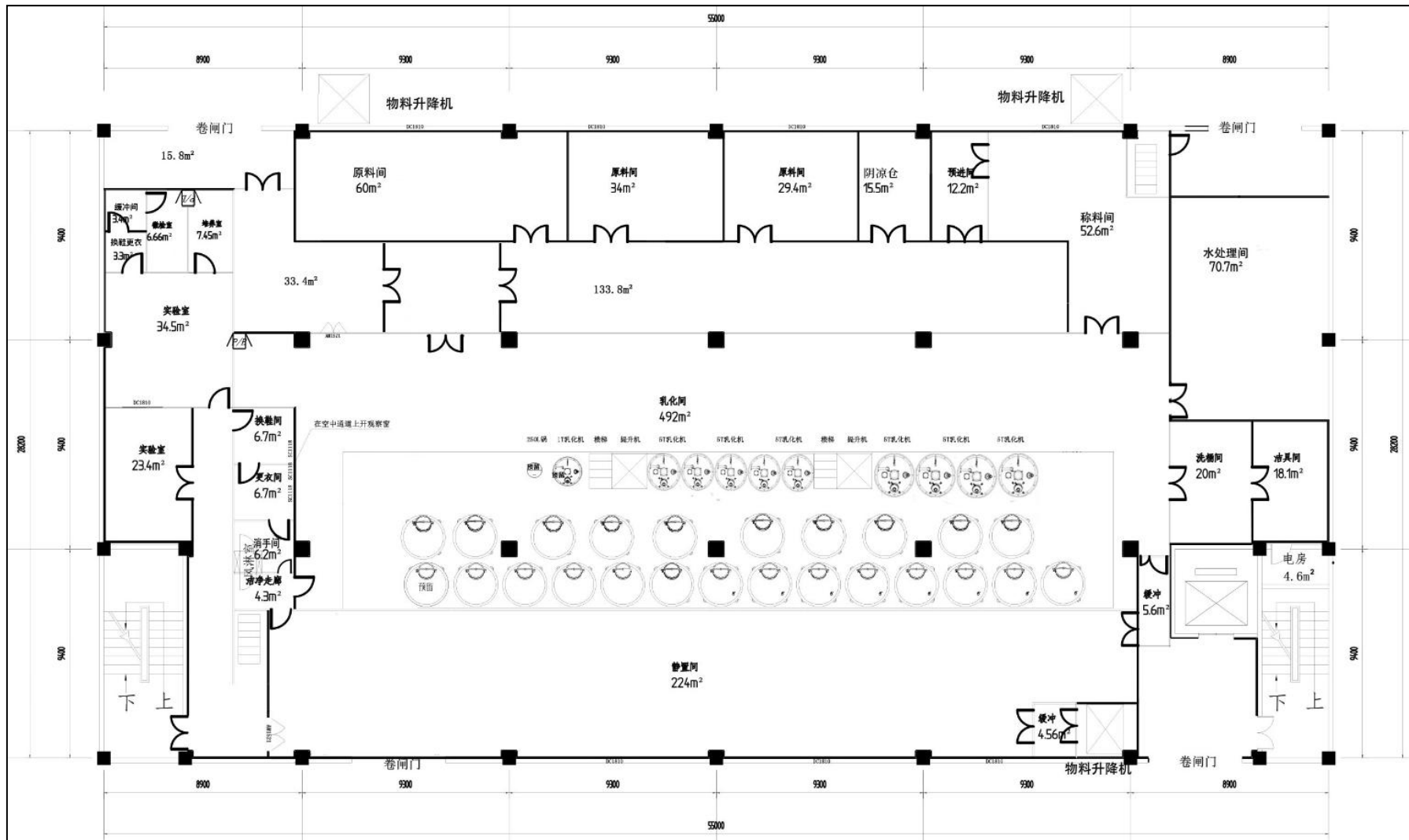
附图 5-1 扩建项目新增厂房一楼
