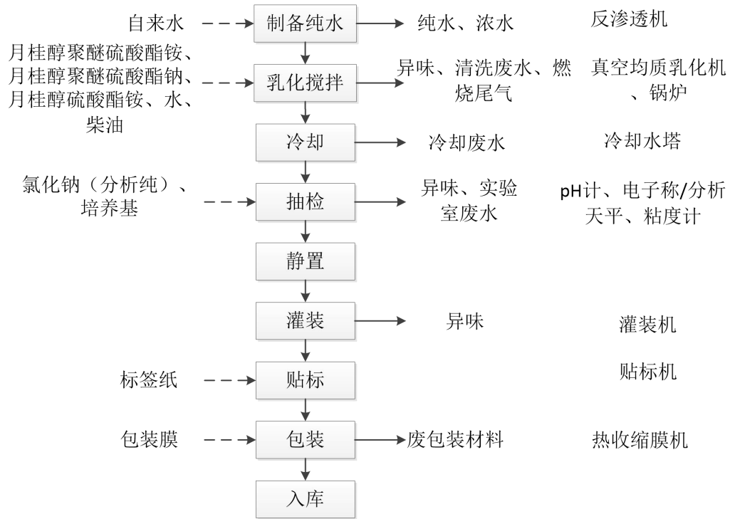
图 2-4 洗发露、沐浴露、护发素和发膜生产工艺
