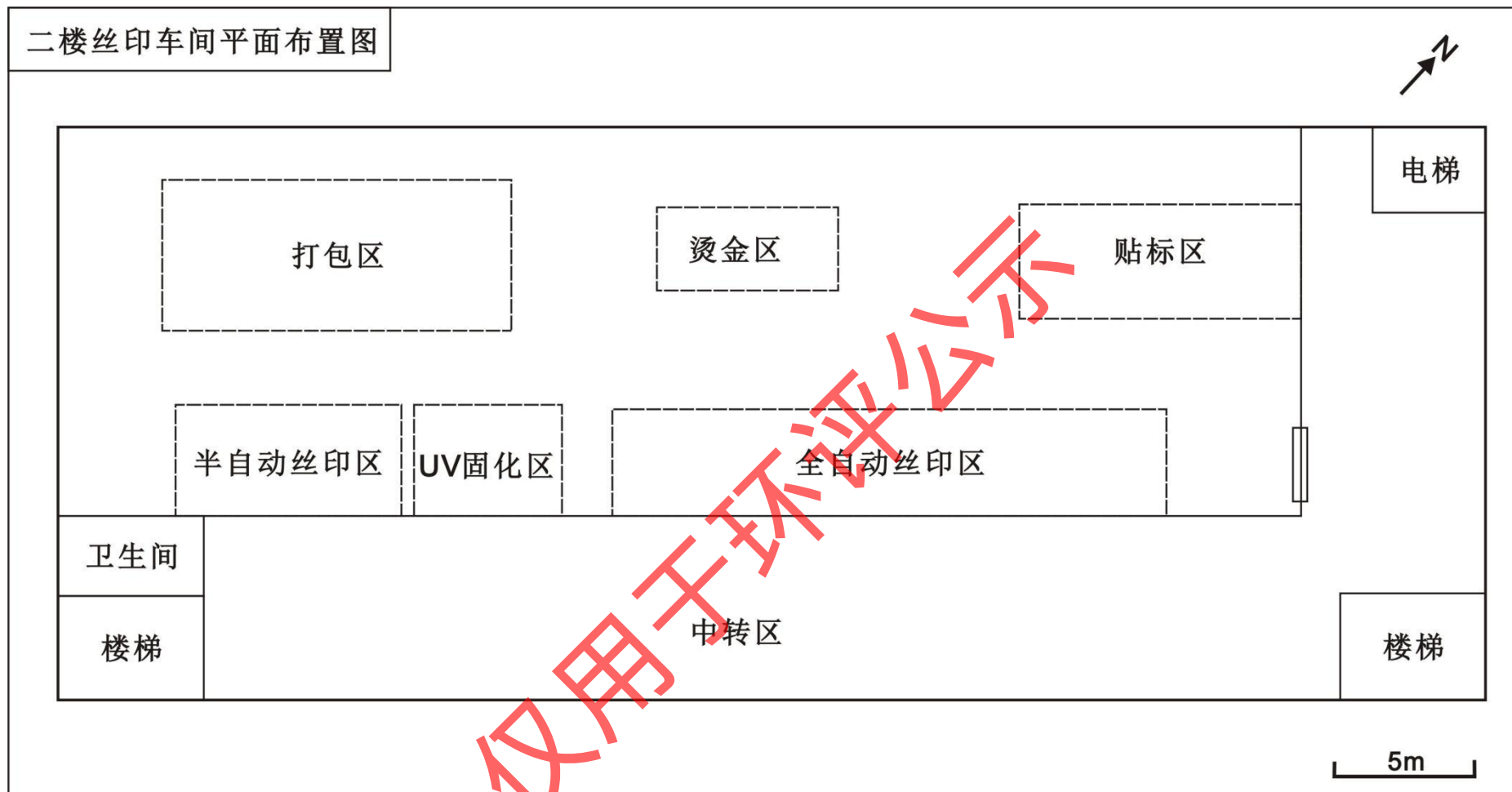
附图 4-2 项目 2 楼丝印车间平面布置图
