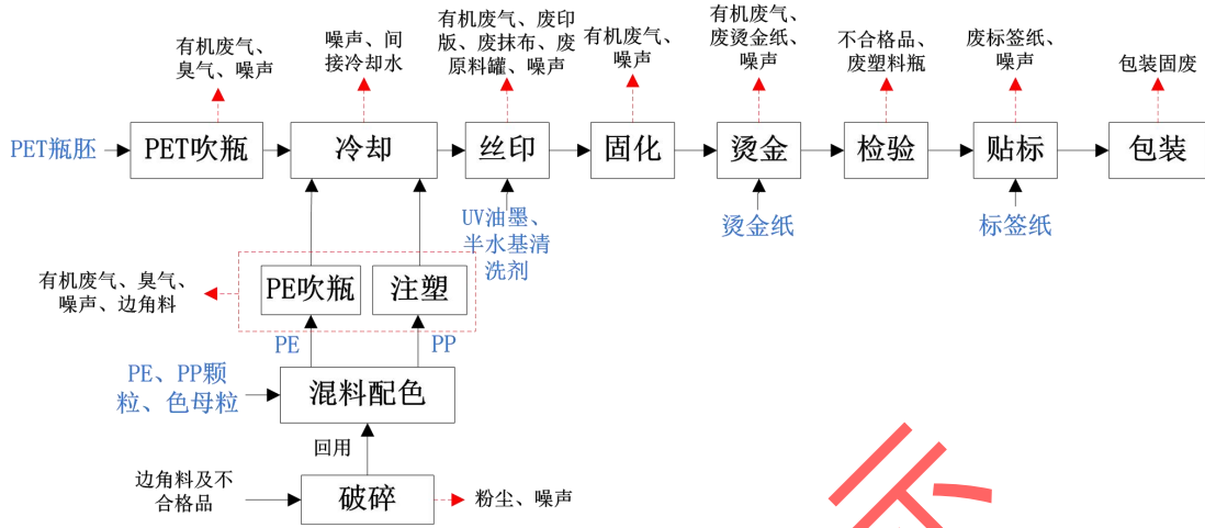
图 2-3 塑料瓶生产工艺流程及产污节点图
