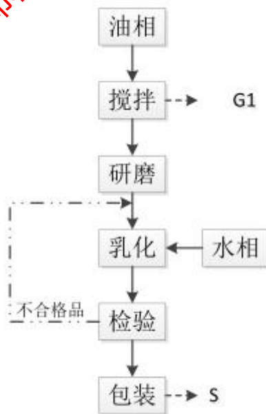
图2-6 迁建前油墨生产工艺流程图
