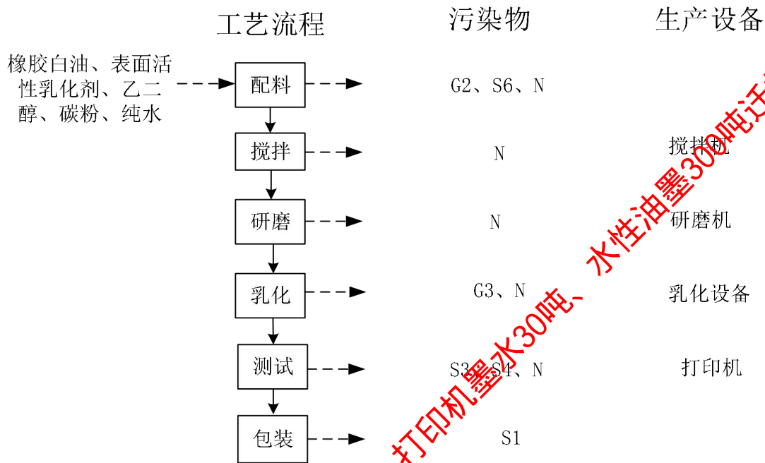
图 2-4 项目水性油墨生产工艺流程图
