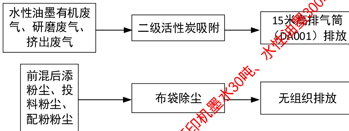
图 4-2 项目废气治理工艺流程图
