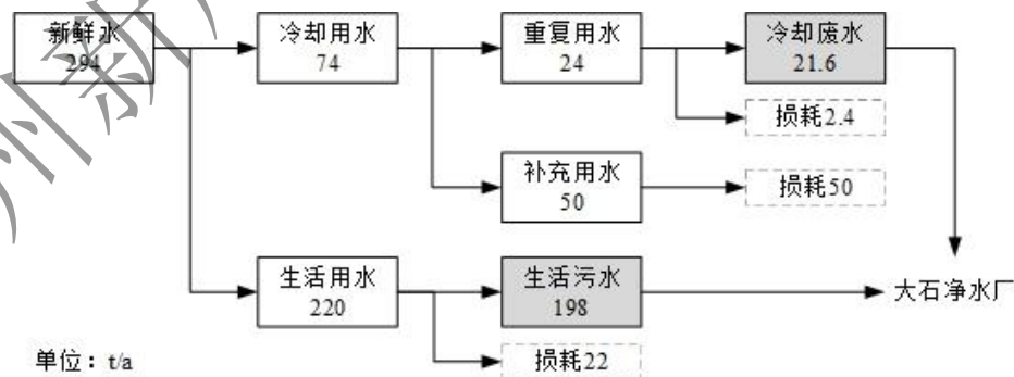
图 2-1 水平衡示意图
