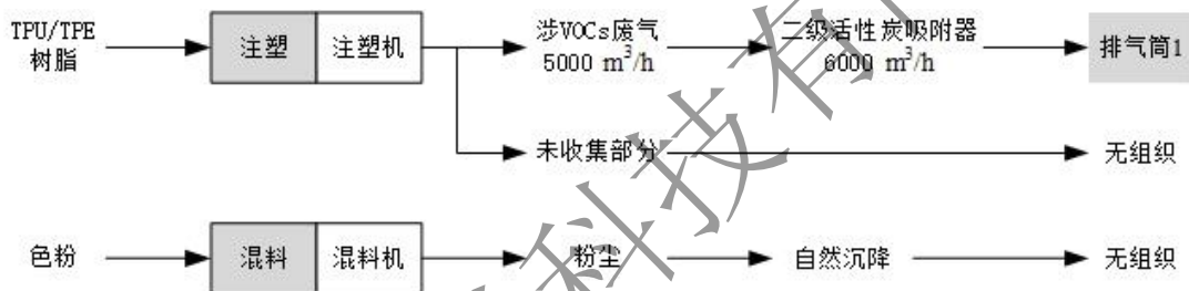
图 4-2 废气收集、治理和排放汇总示意图
