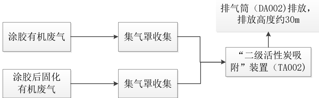
图 4-1 项目涂胶、涂胶后固化有机废气处理工艺流程图
