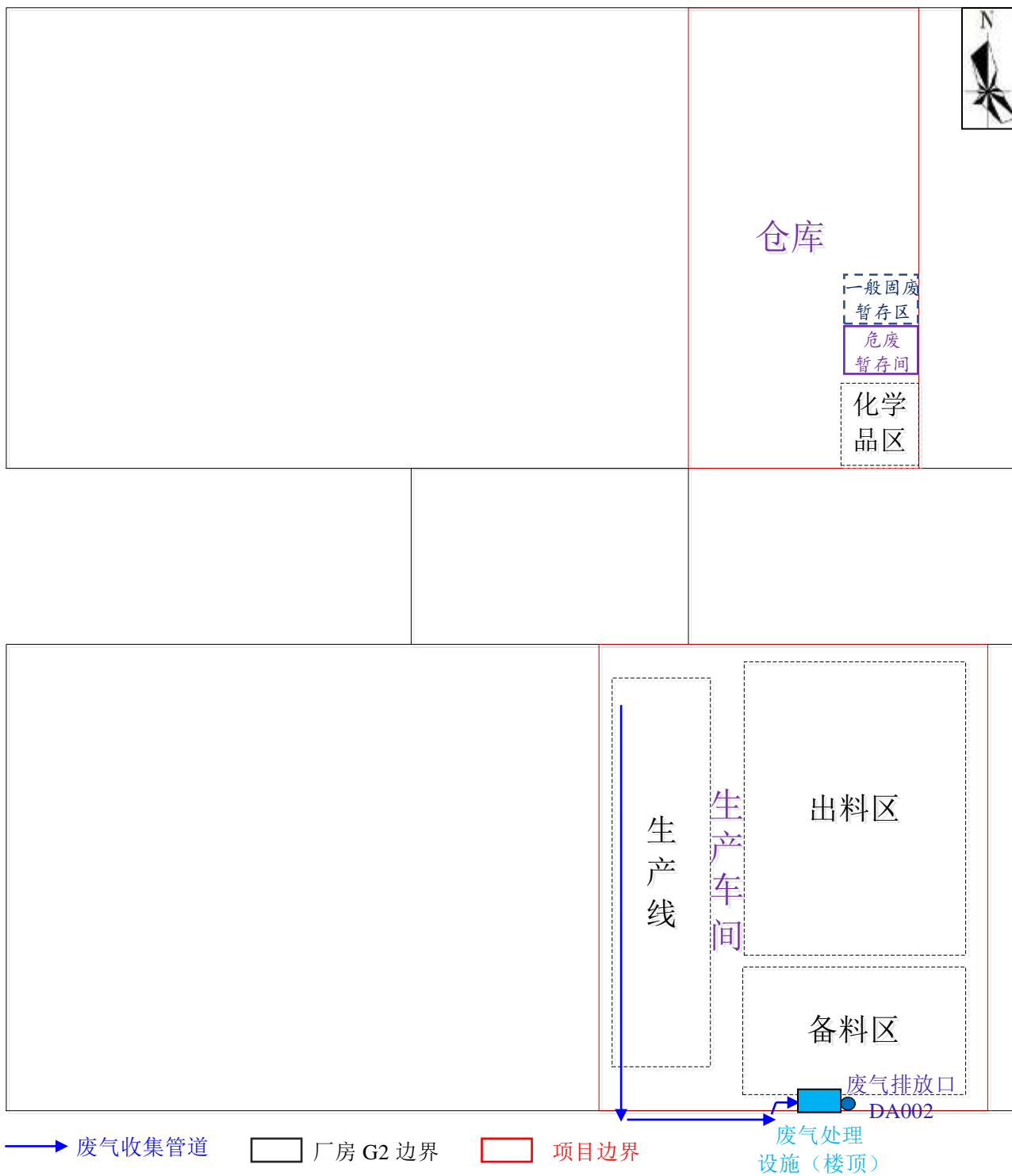
项目平面布置图
