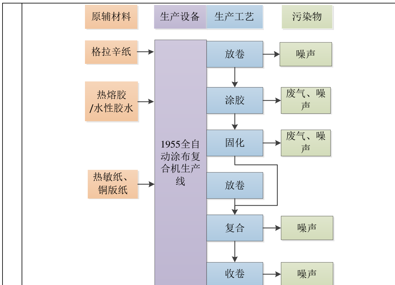
图2-2 项目生产工艺流程及产污环节图
