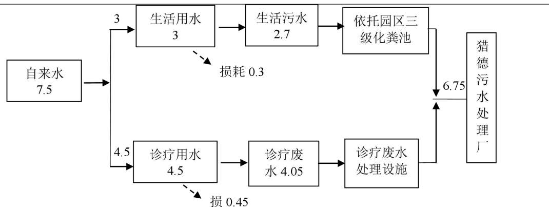
图 2-1 扩建项目水平衡图 单位: m^3/a
