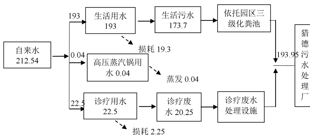
图 2-2 扩建后总体项目水平衡图 单位: m^3/a
