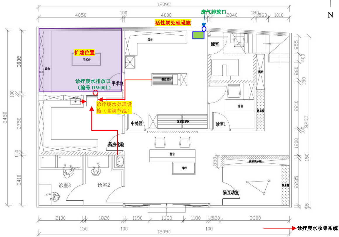
首层平面图
