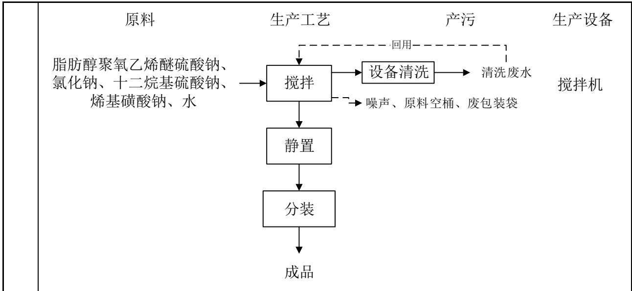
图 2-8 原项目泡沫剂生产工艺流程图
