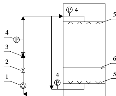
1-冲洗水泵 2-调节阀 3-流量计 4-压力表 5-喷嘴 6-水量分布测定装置
