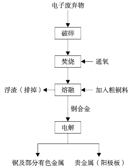
图 3 火法冶金工艺流程
