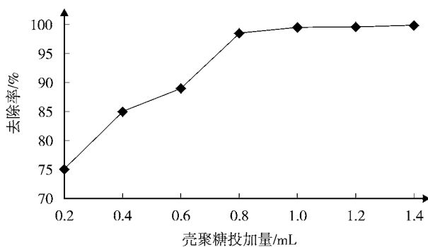
图 3 壳聚糖投加量对 Pb^{2+} 去除率的影响
