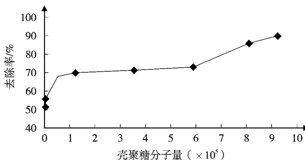
图 1 不同分子量壳聚糖对 Pb^{2+} 去除率的影响
