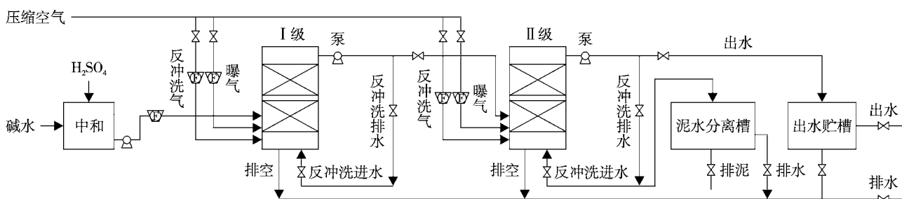
图 1 BAF 工艺流程
