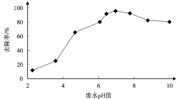
图 4 不同 pH 值对 Pb^{2+} 去除率的影响
