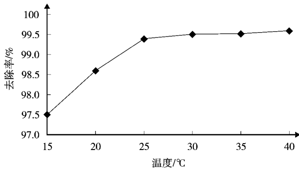
图5 温度对 Pb 2+ 去除率的影响
