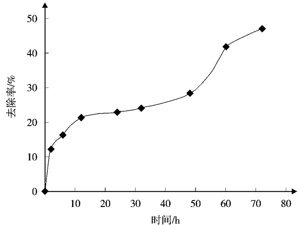
图 4 总磷去除率变化
