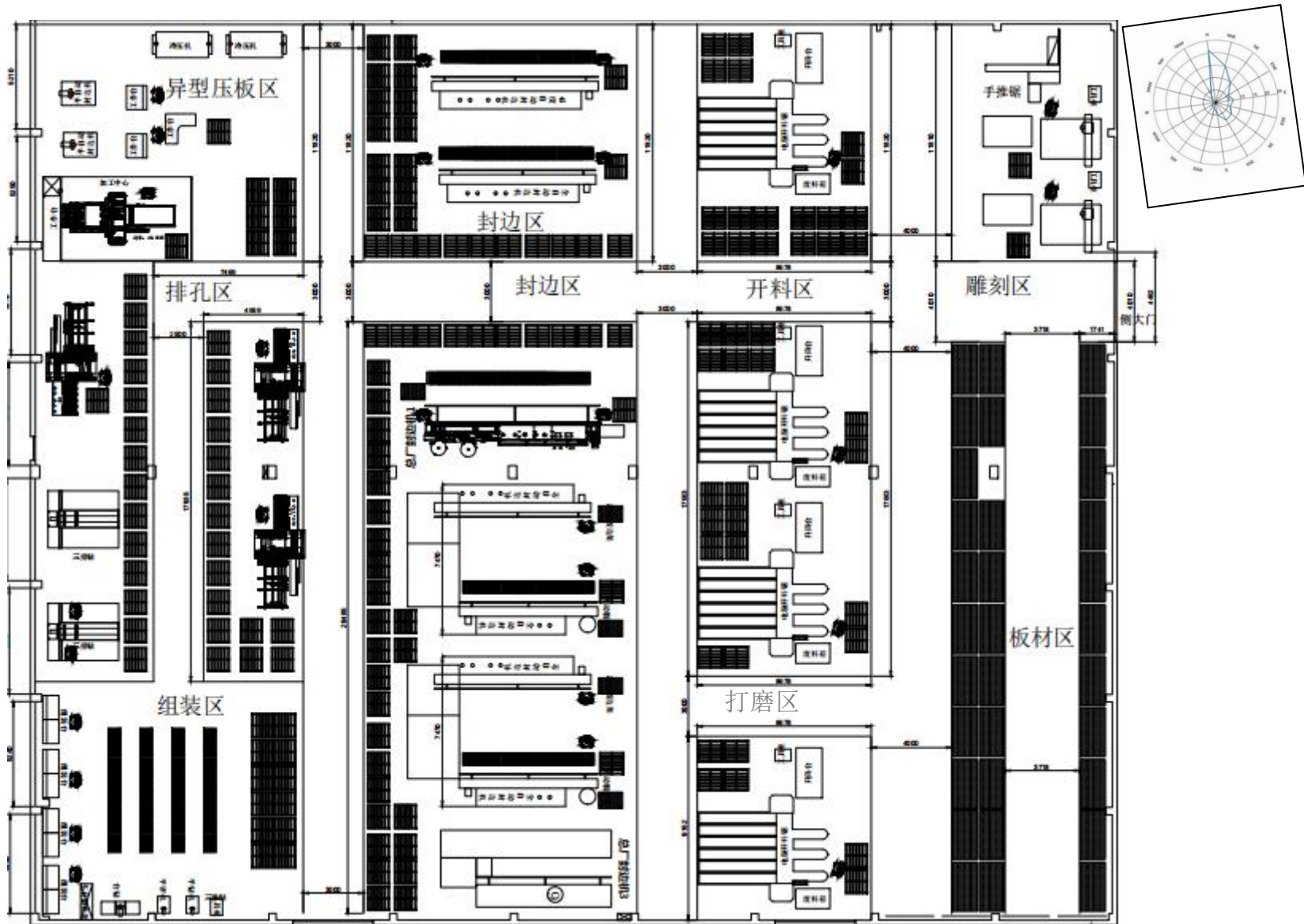
附图 5-2 项目车间 1 平面图
