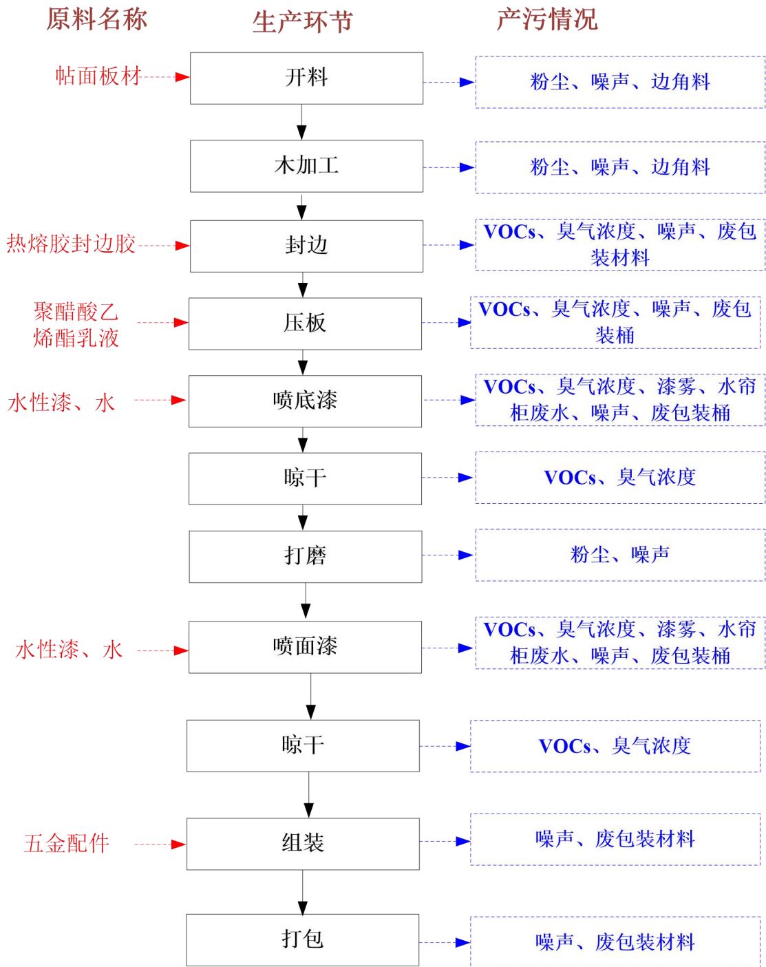
图 2-2 工艺流程图
