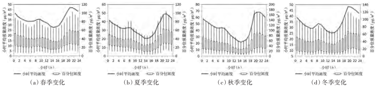
图4 NO 2 的小时值变化趋势
