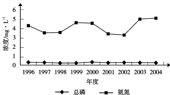
图 1 1996~2004 年珠江黄沙河段水质总磷和氨氮的变化
